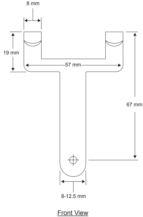
Dwg. 3
