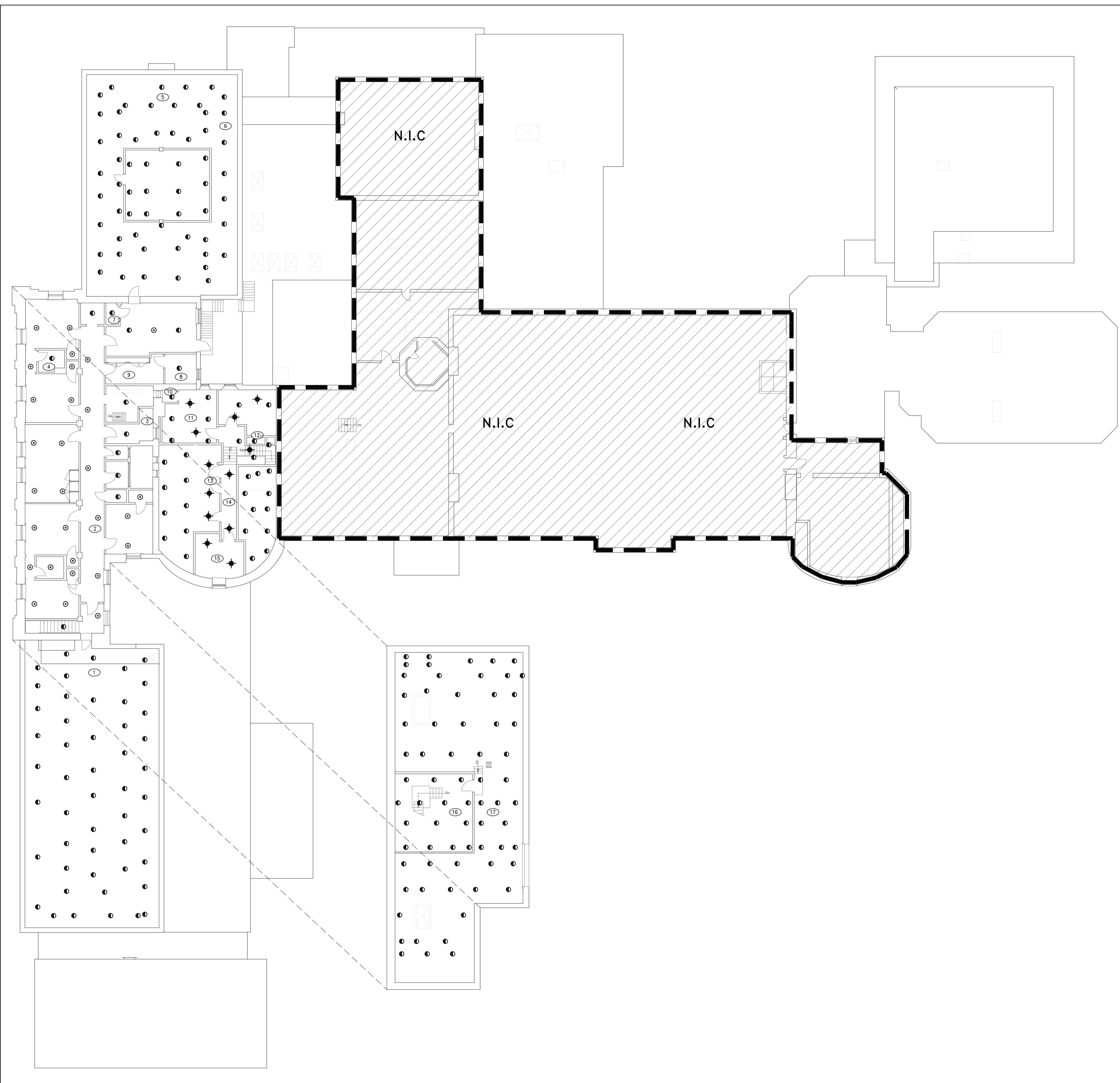
1 FP4 NEW THIRD FLOOR SPRINKLERS LAYOUT TROISIEME ÉTAGES - NOUVELLE EMPLACEMENT DES GICLEURS SCALE/ÉCHELLE 1 : 175
