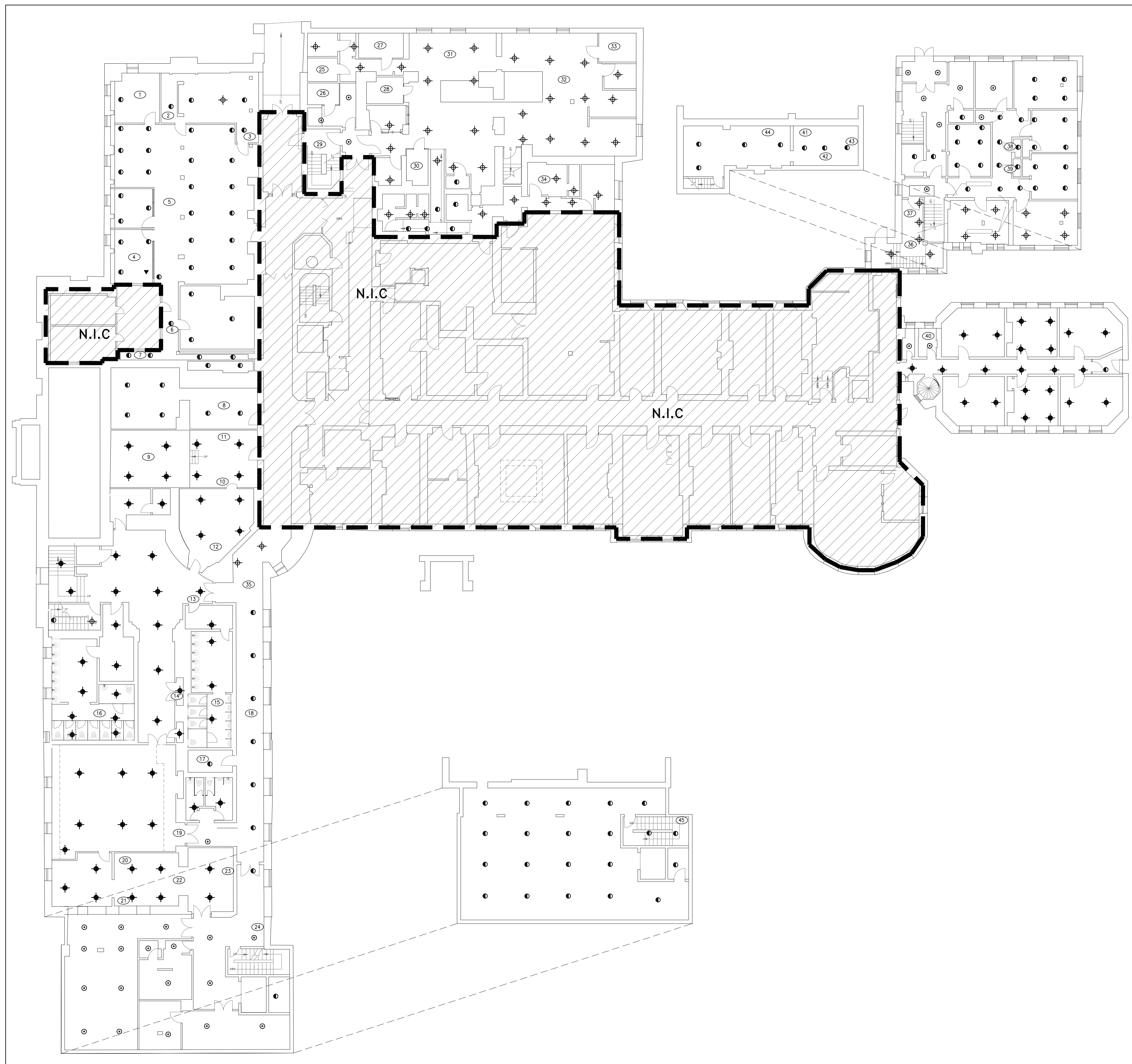
1 NEW BASEMENT SPRINKLERS LAYOUT SOUS-SOL - NOUVELLE EMPLACEMENT DES GICLEURS SCALE/ÉCHELLE: 1 : 175
