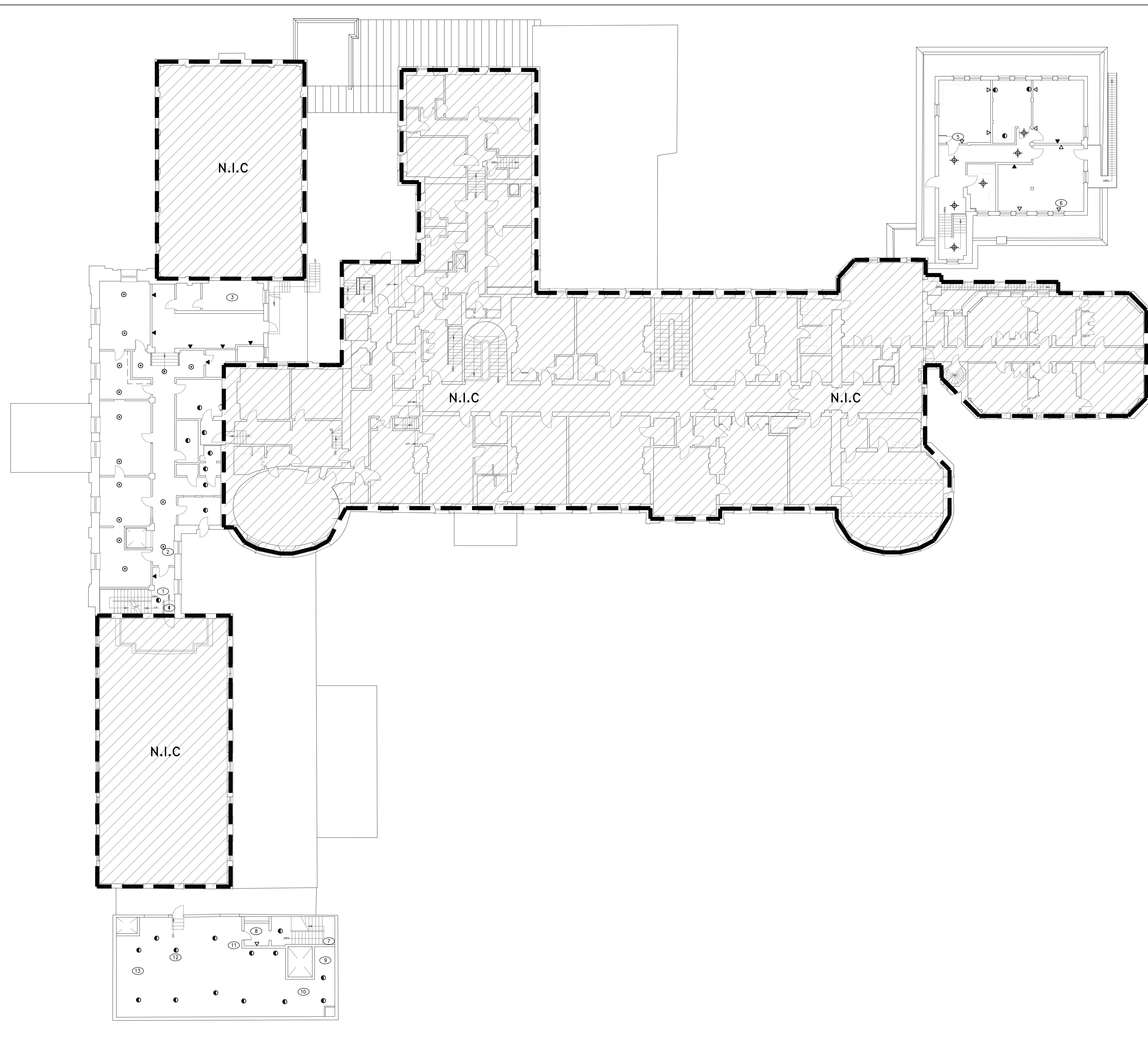
1 NEW SECOND FLOOR SPRINKLERS LAYOUT FP3 DEUXIEME ÉTAGES - NOUVELLE EMPLACEMENT DES GICLEURS SCALE/ÉCHELLE 1 : 175
