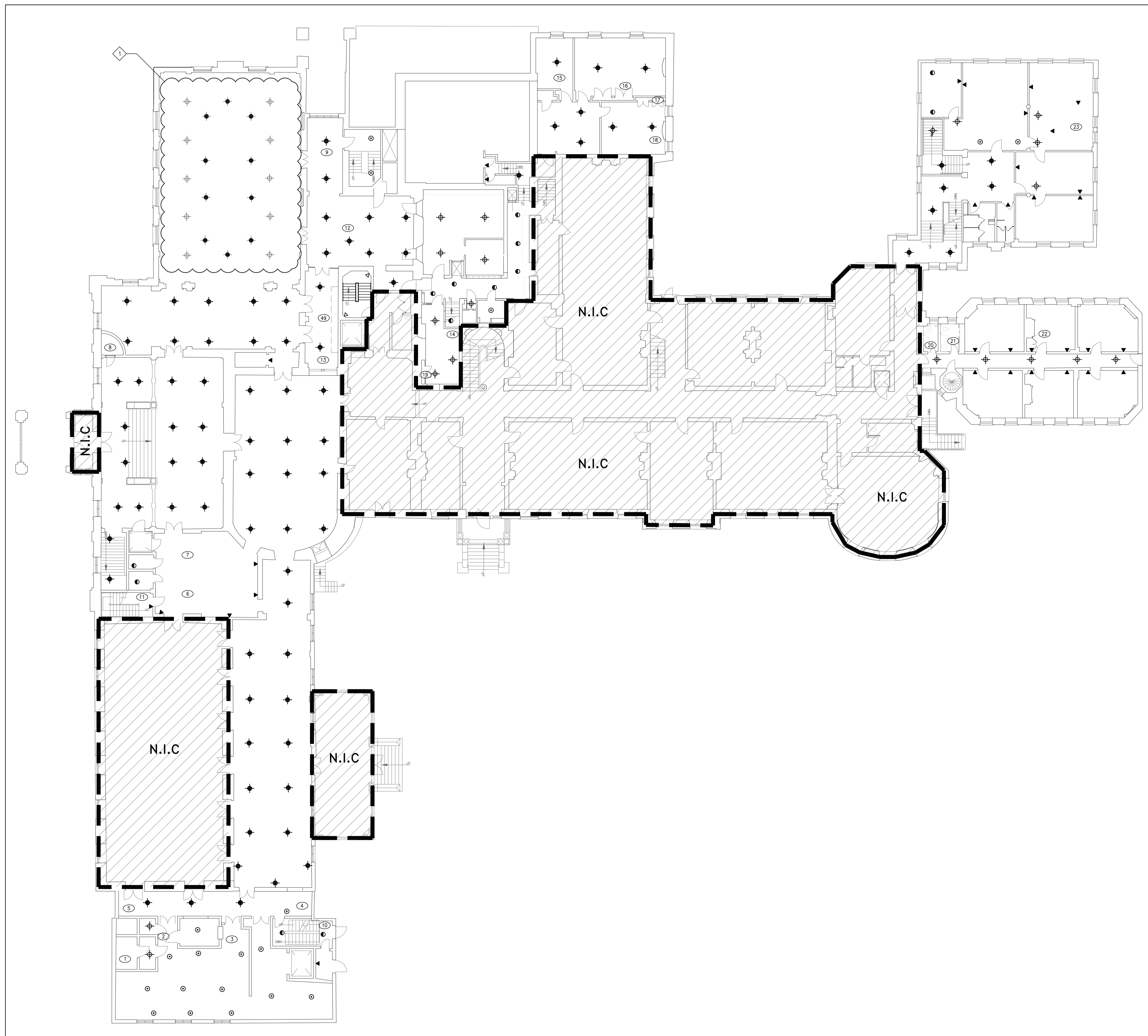
1 NEW GROUND FLOOR SPRINKLERS LAYOUT FP2 REZ-DE-CHAUSSÉ - NOUVELLE EMLACEMENT DES GICLERS SCALE/ÉCHELLE 1 : 175
