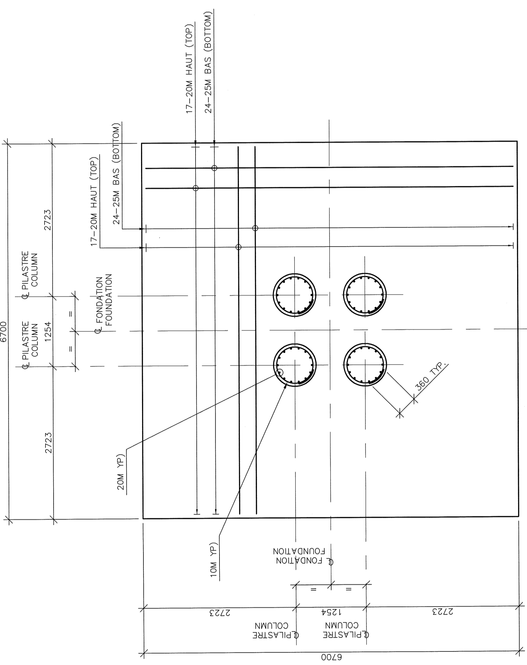
FONDATION— VUE EN PLAN FOUNDATION— PLAN VIEW (1:40)
