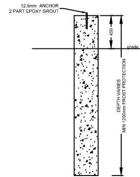
2 201 PIER DETAIL SCALE: 1:20
