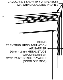
2 WALL DETAILS 302 SCALE: 1:20
