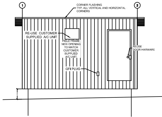
2 NORTH ELEVATION 301 SCALE: 1:20
