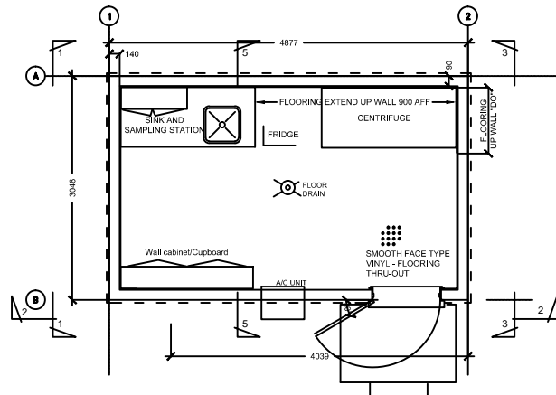
4 FLOOR PLAN 301 SCALE: 1:20
