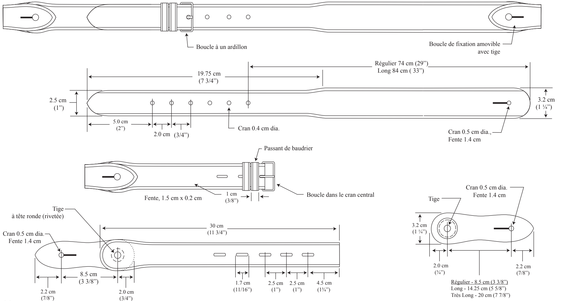
Détails de la sangle pour boucle
