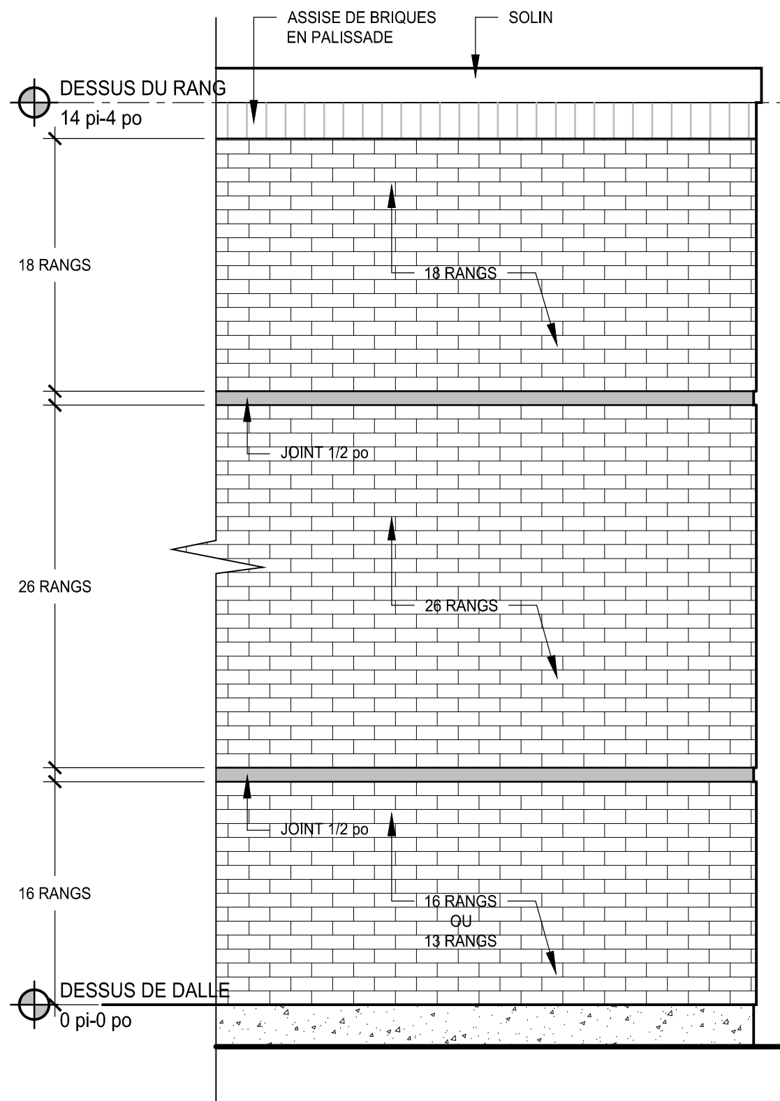
1 ÉLÉVATION DE L'APPAREIL ÉCHELLE : NON À L'ÉCHELLE
