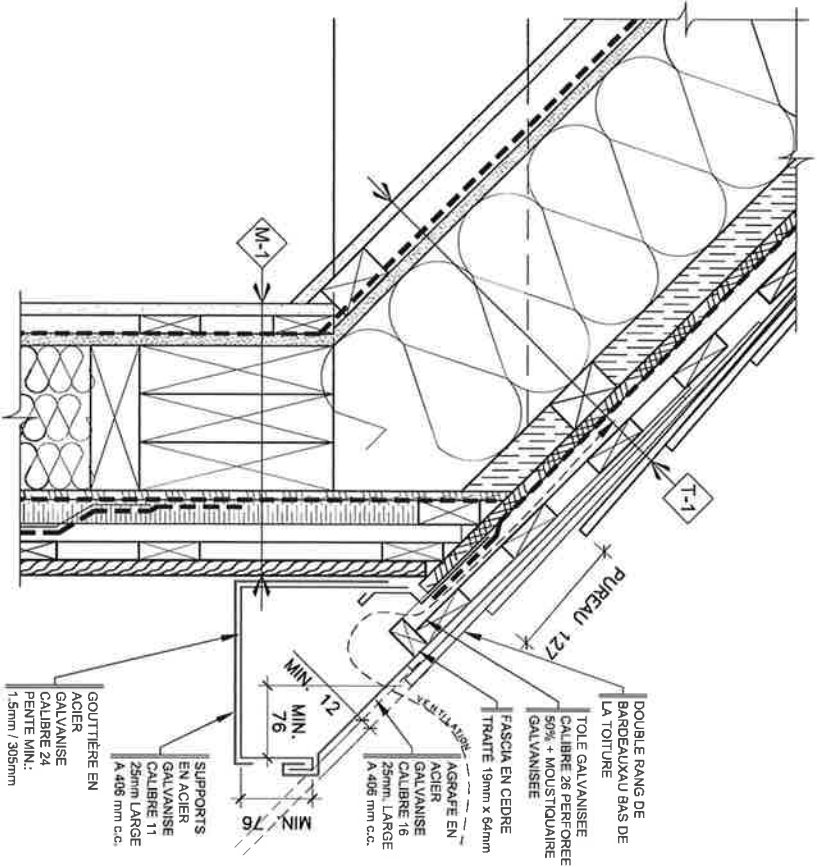
B DÉTAIL GOUTTIÈRE ET FASCIA 06 11 ECHELLE: 1:5
