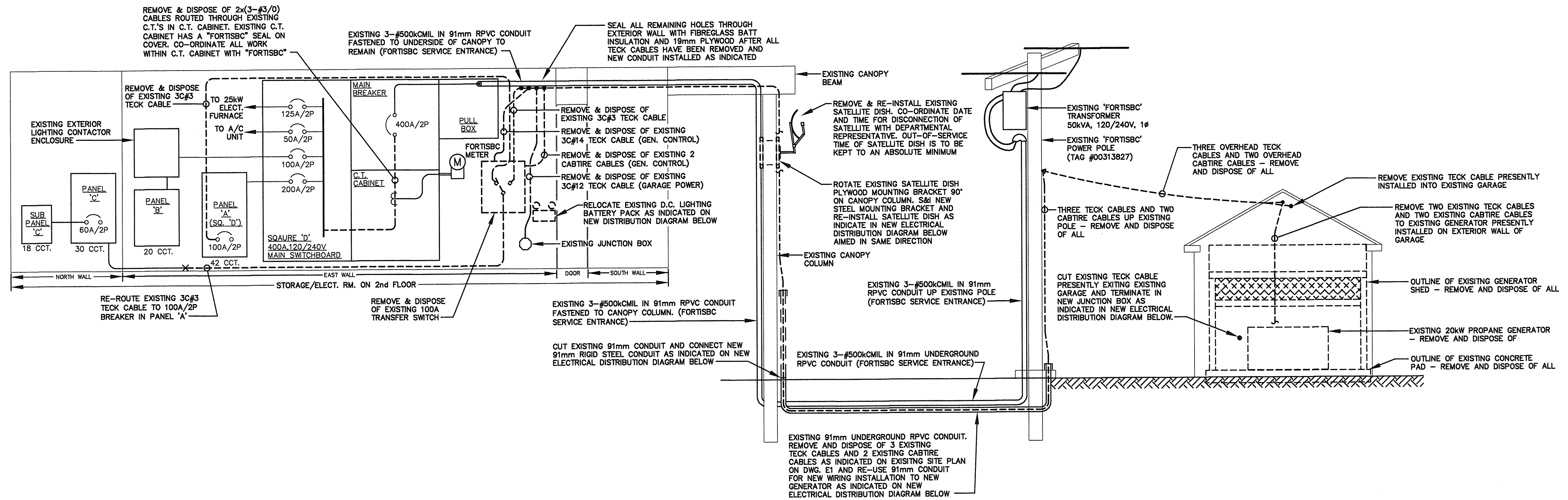
EXISTING ELECTRICAL DISTRIBUTION DIAGRAM SCALE: N.T.S.
