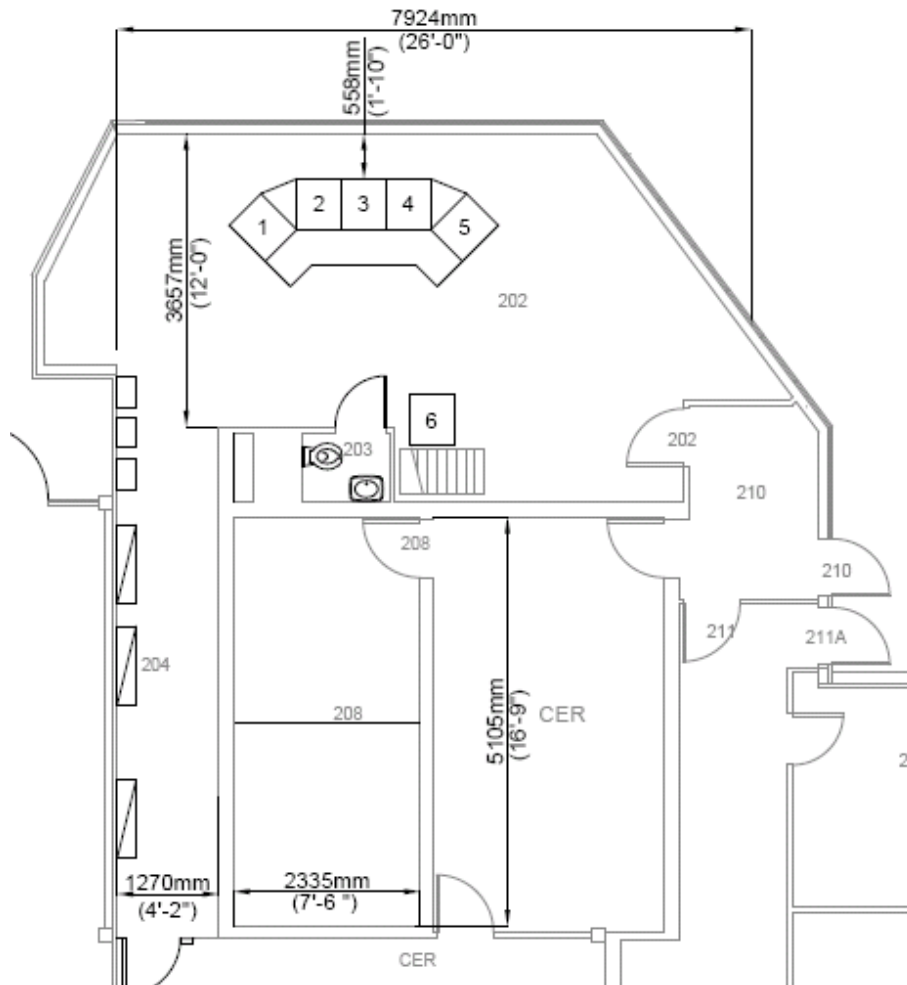
Figure 1 : Aménagement des baies et de l'armoire de la console du PPCC existant
