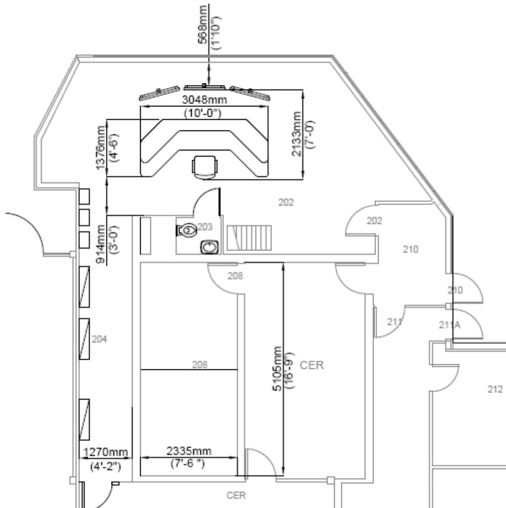
Figure 2 : Emplacement de la nouvelle console du PPCC
