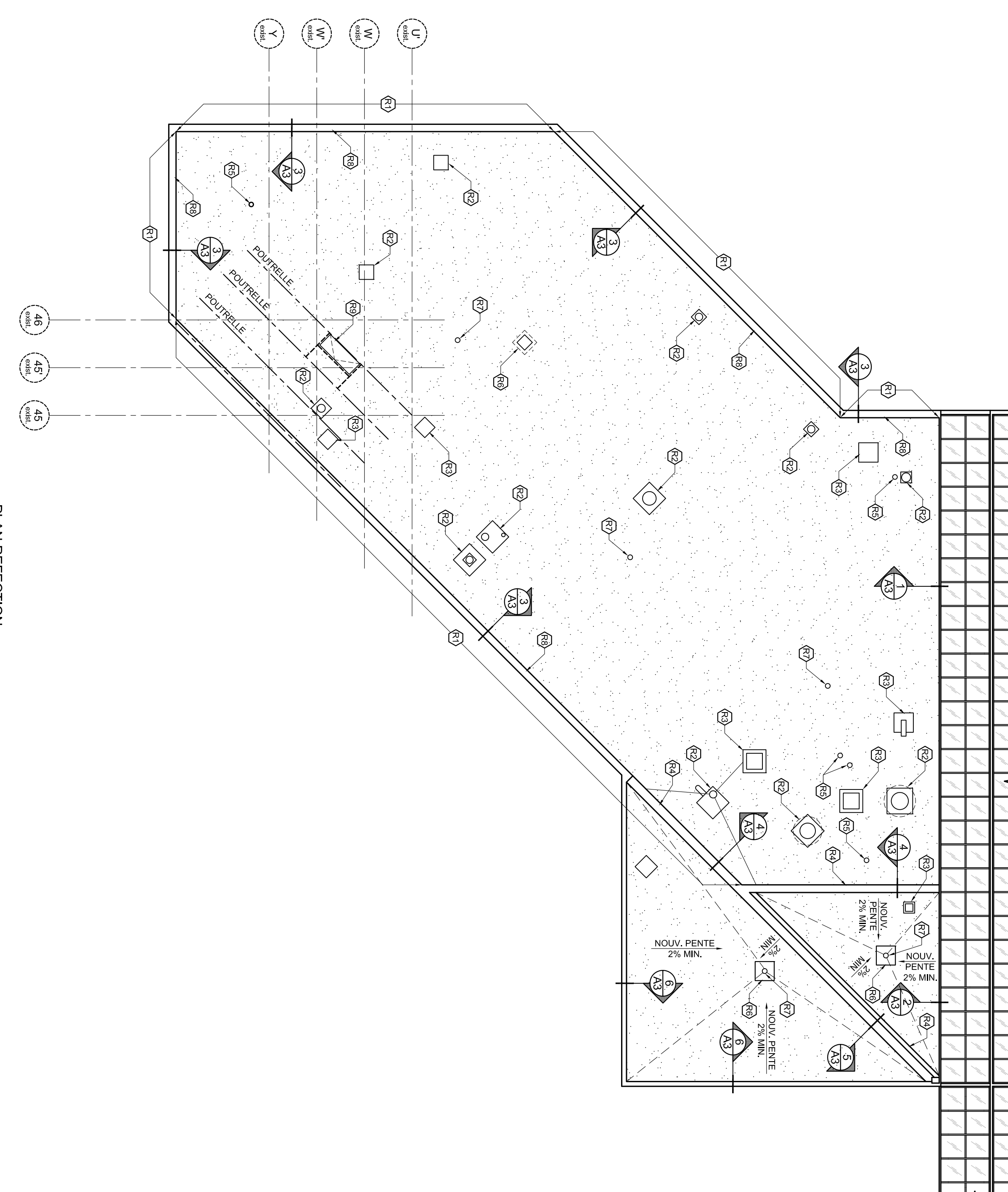
PLAN REFECTION TOITURE SECTEUR 1, 2 ET 3 ÉCHELLE: 1:300
