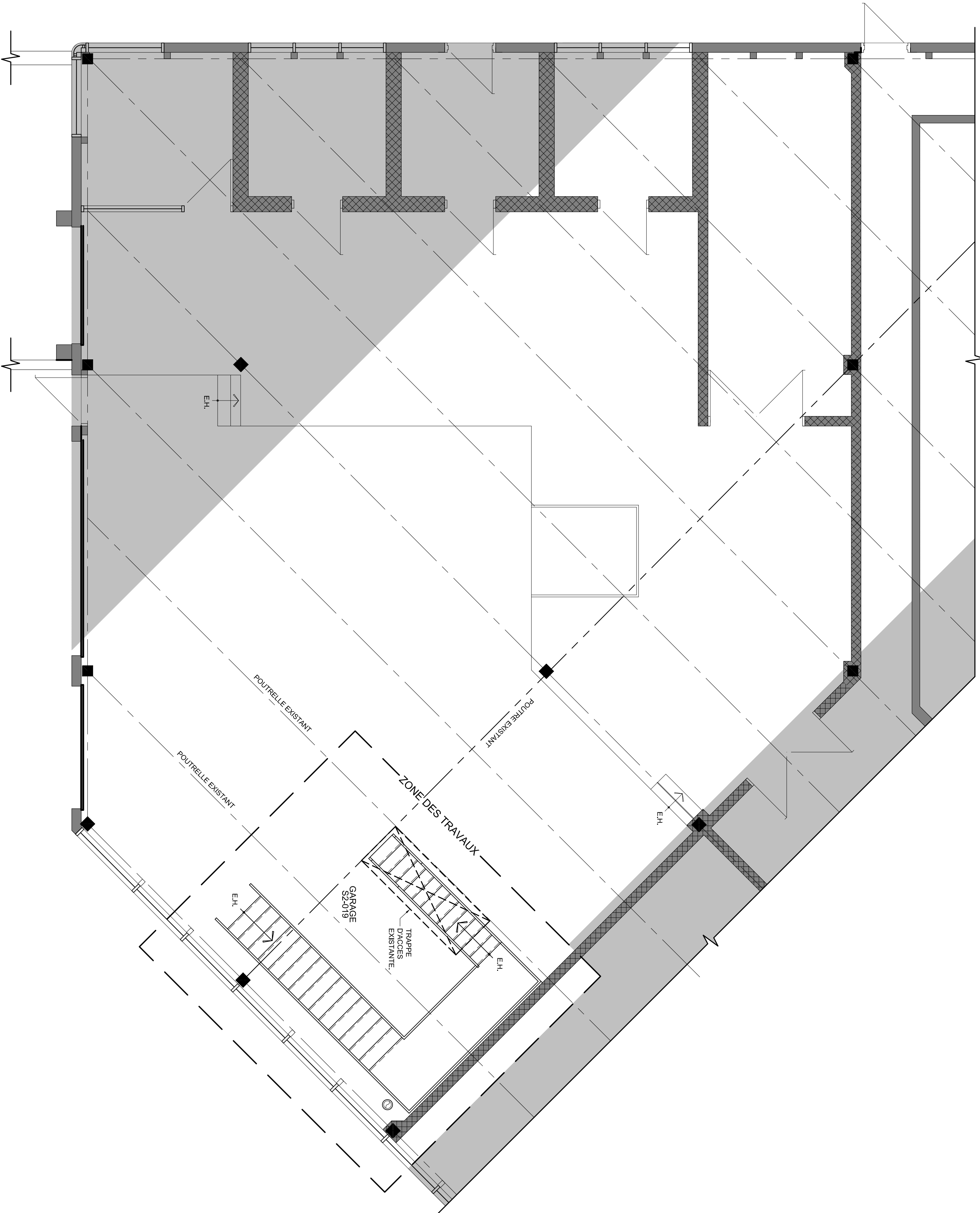
PLAN D'AMÉNAGEMENT D'UNE NOUVELLE ESCALIER ÉCHELLE : 1:50
