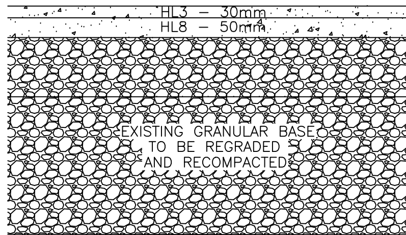
NEW PAVEMENT SECTION N.T.S.
