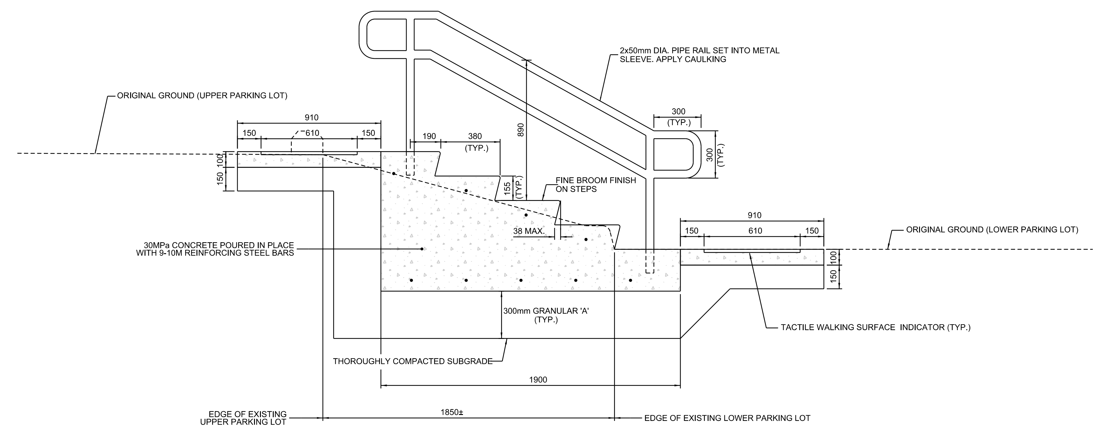
SECTION D-D 1:15
