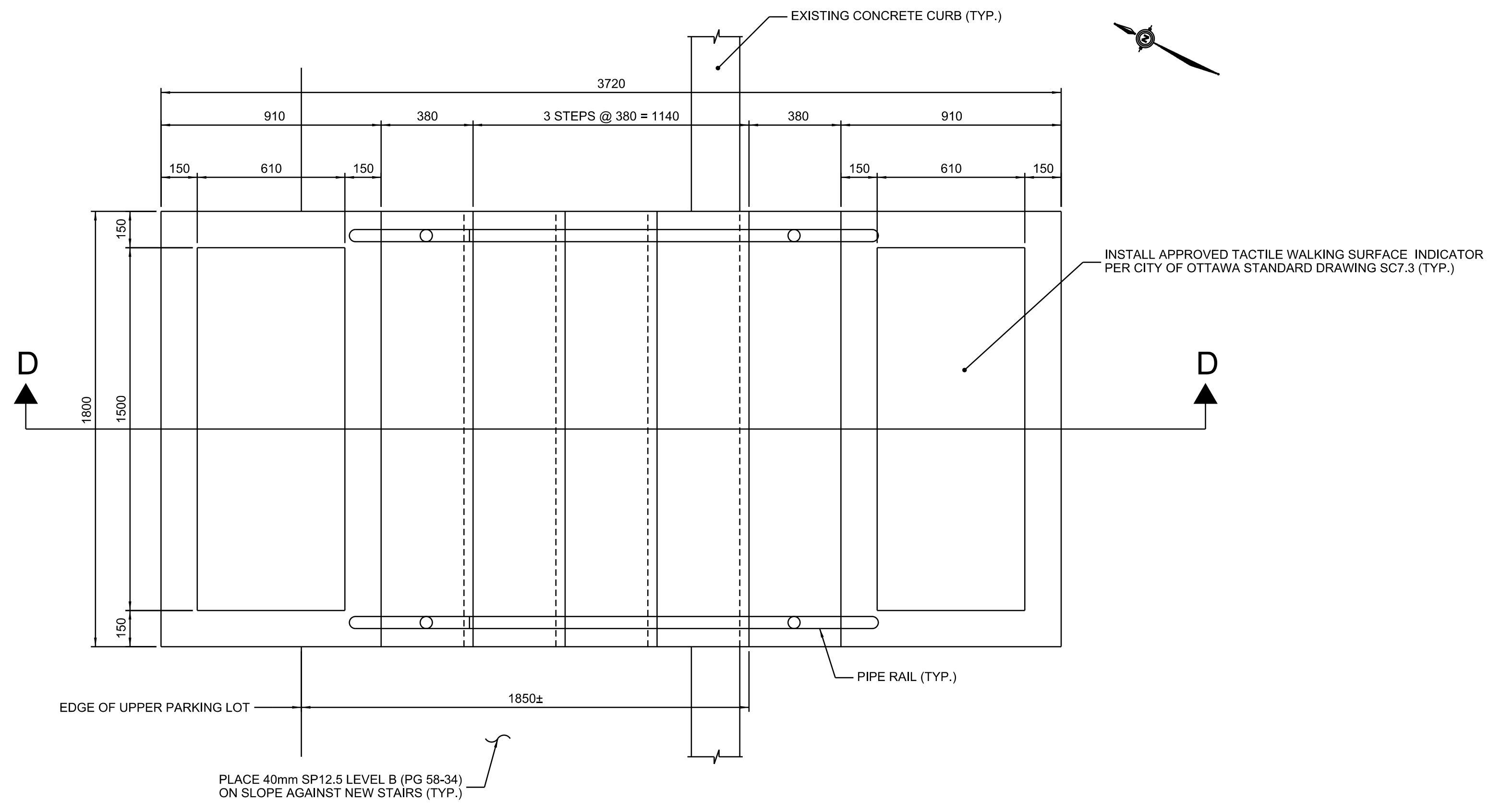
PLAN 1:15
