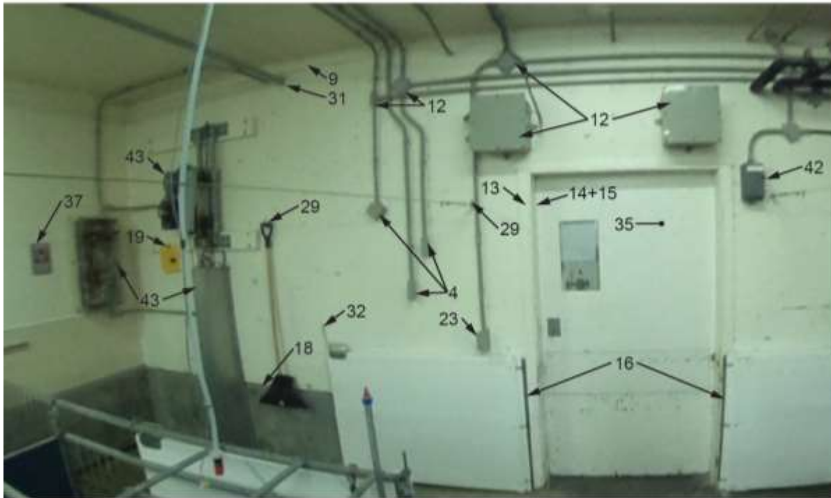
Élévation 1
