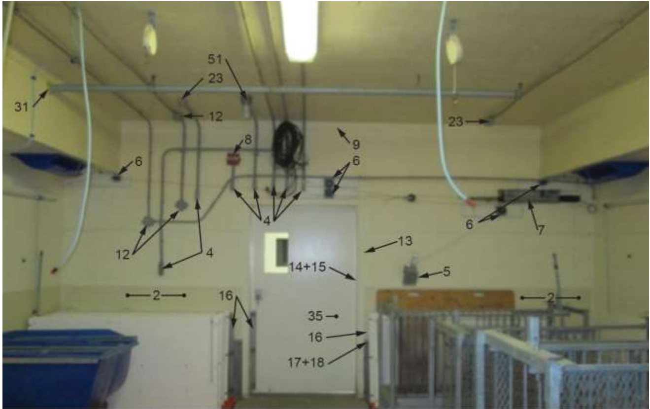
Élévation 1
