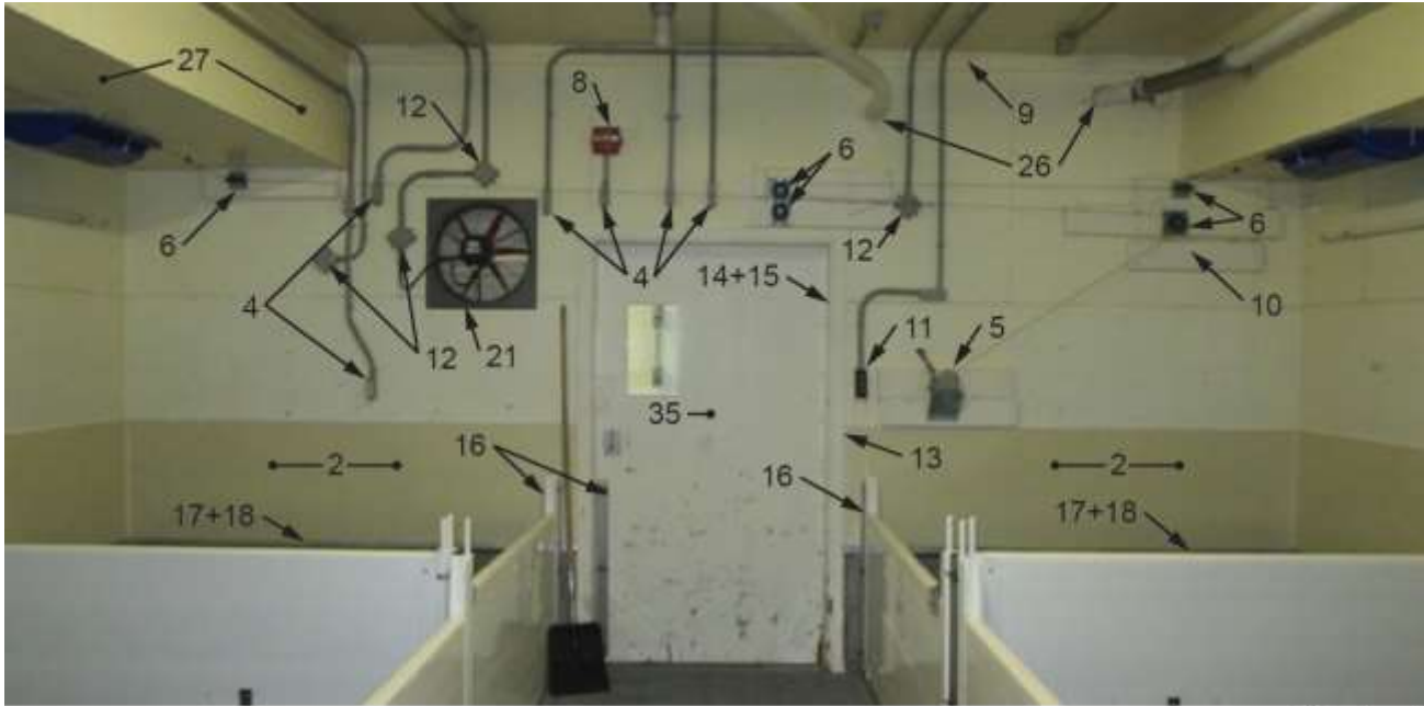
Élévation 1
