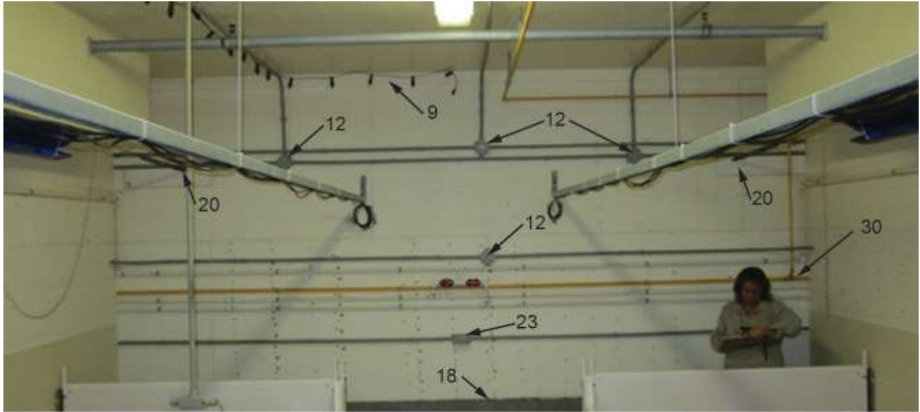
Élévation 3
