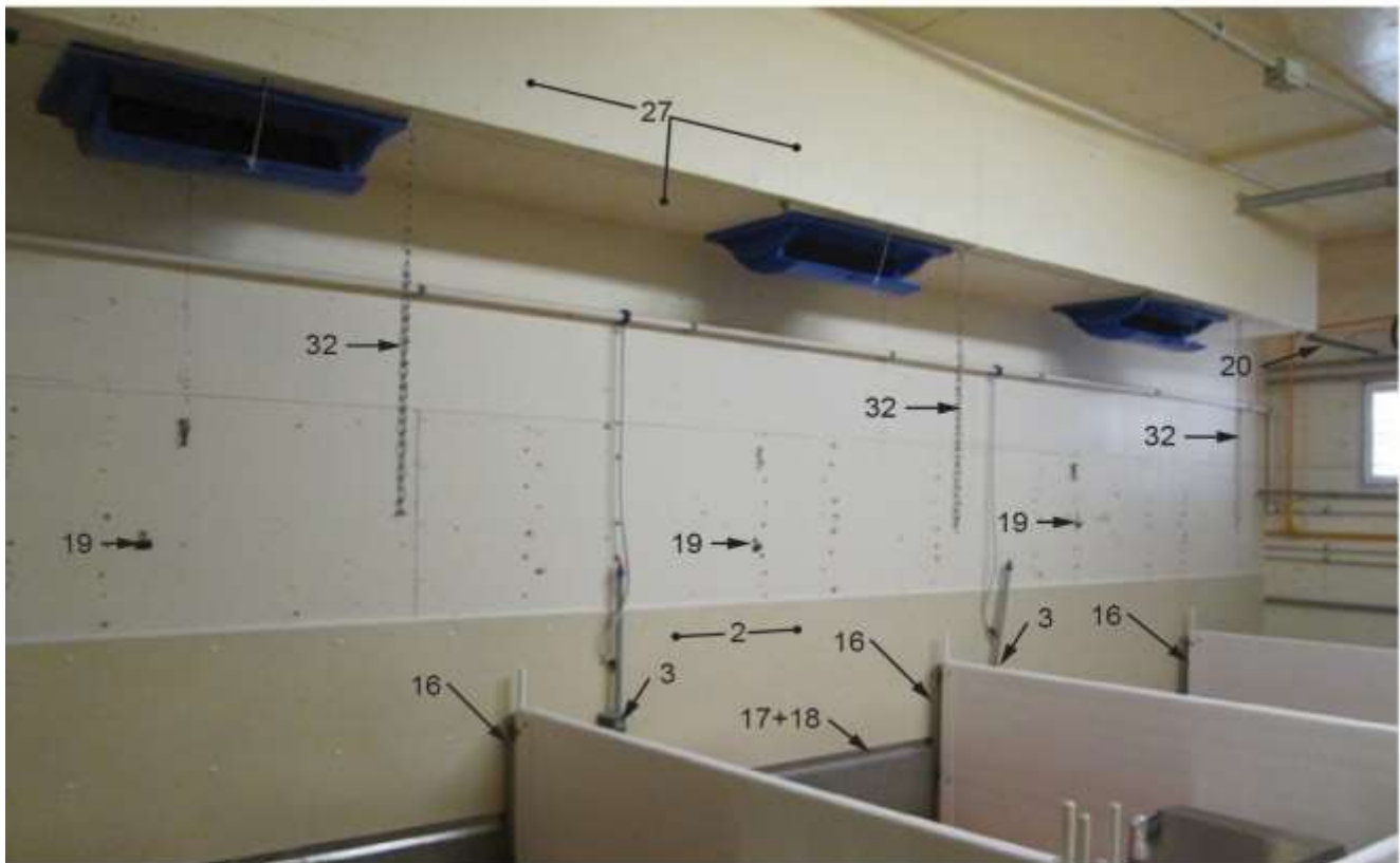
Élévation 2
