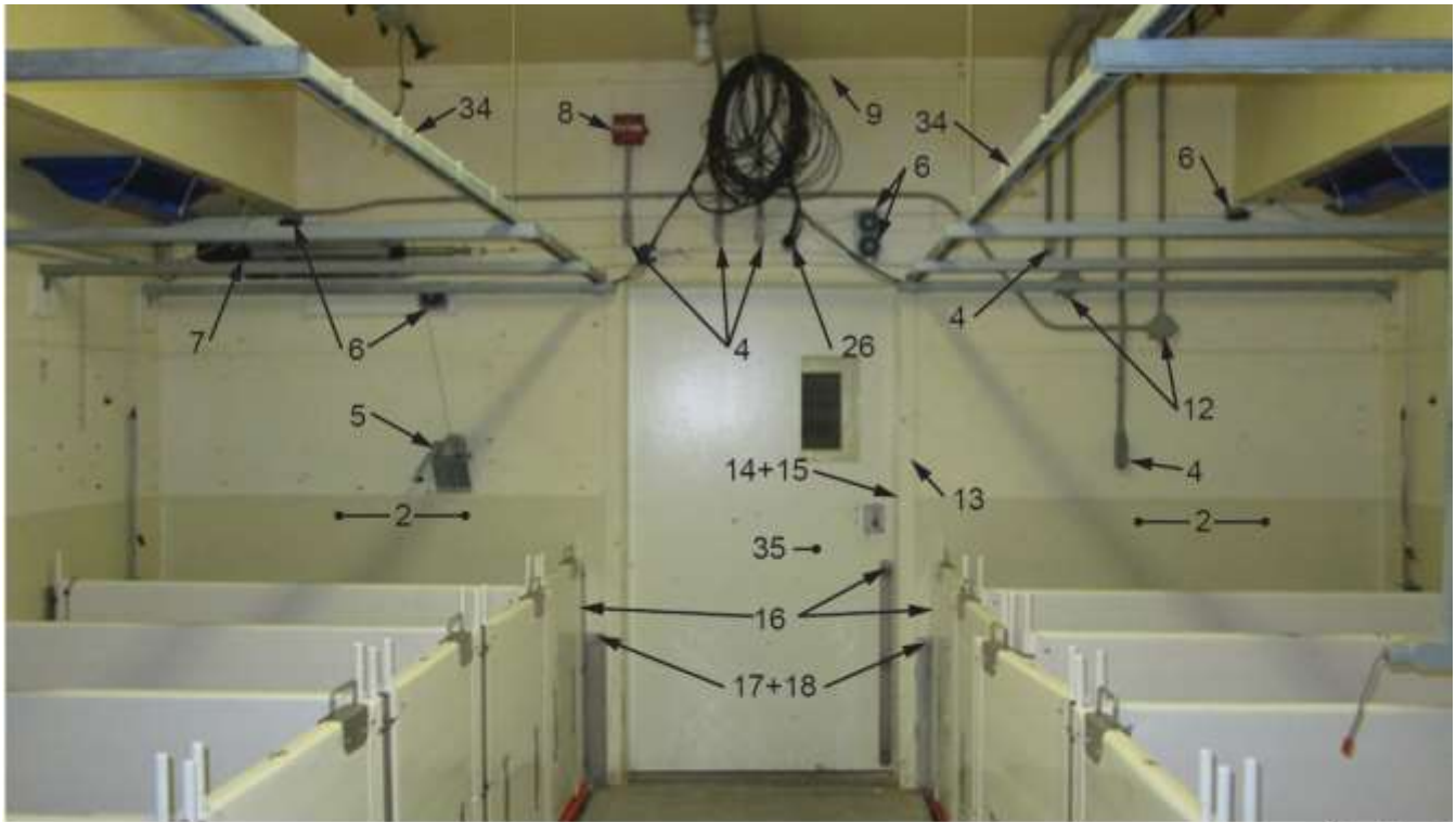
Élévation 1
