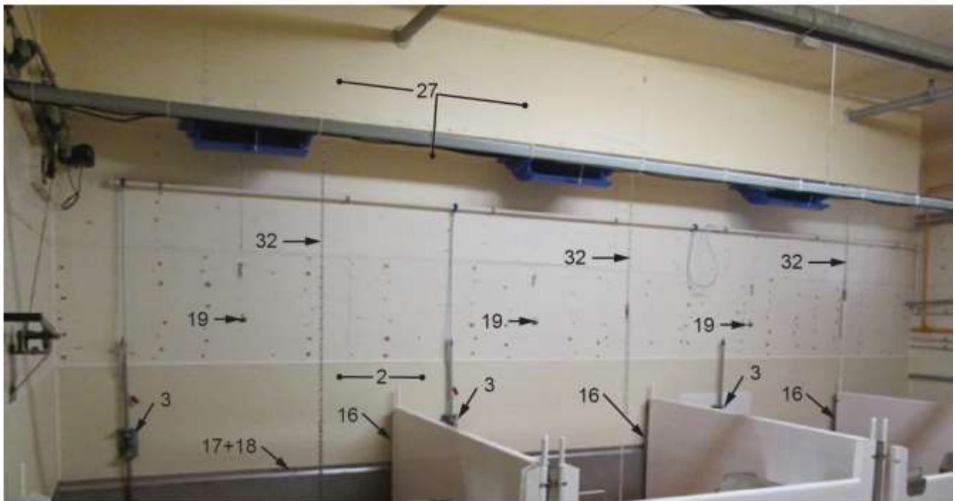
Élévation 2
