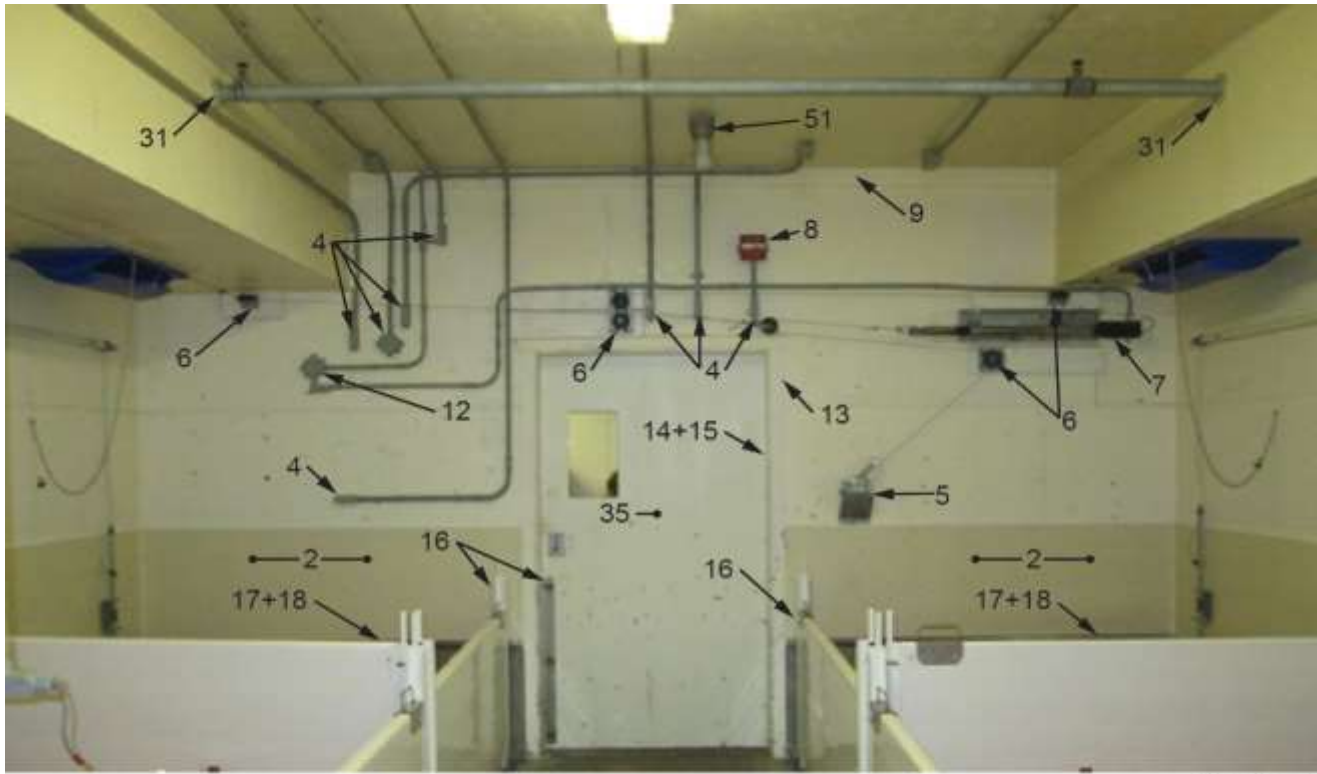
Élévation 1
