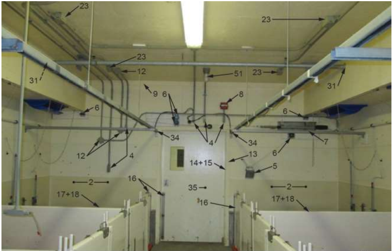
Élévation 1
