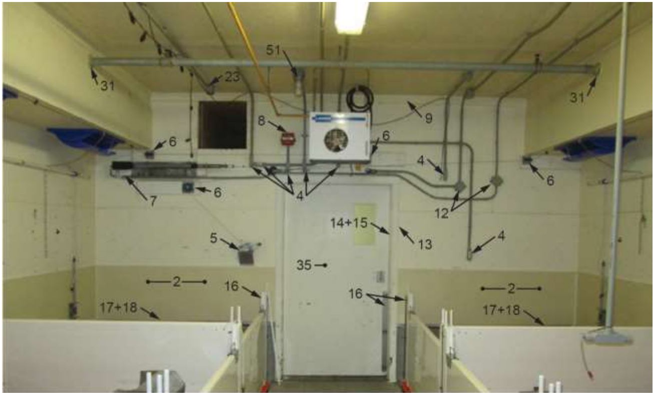
Élévation 1
