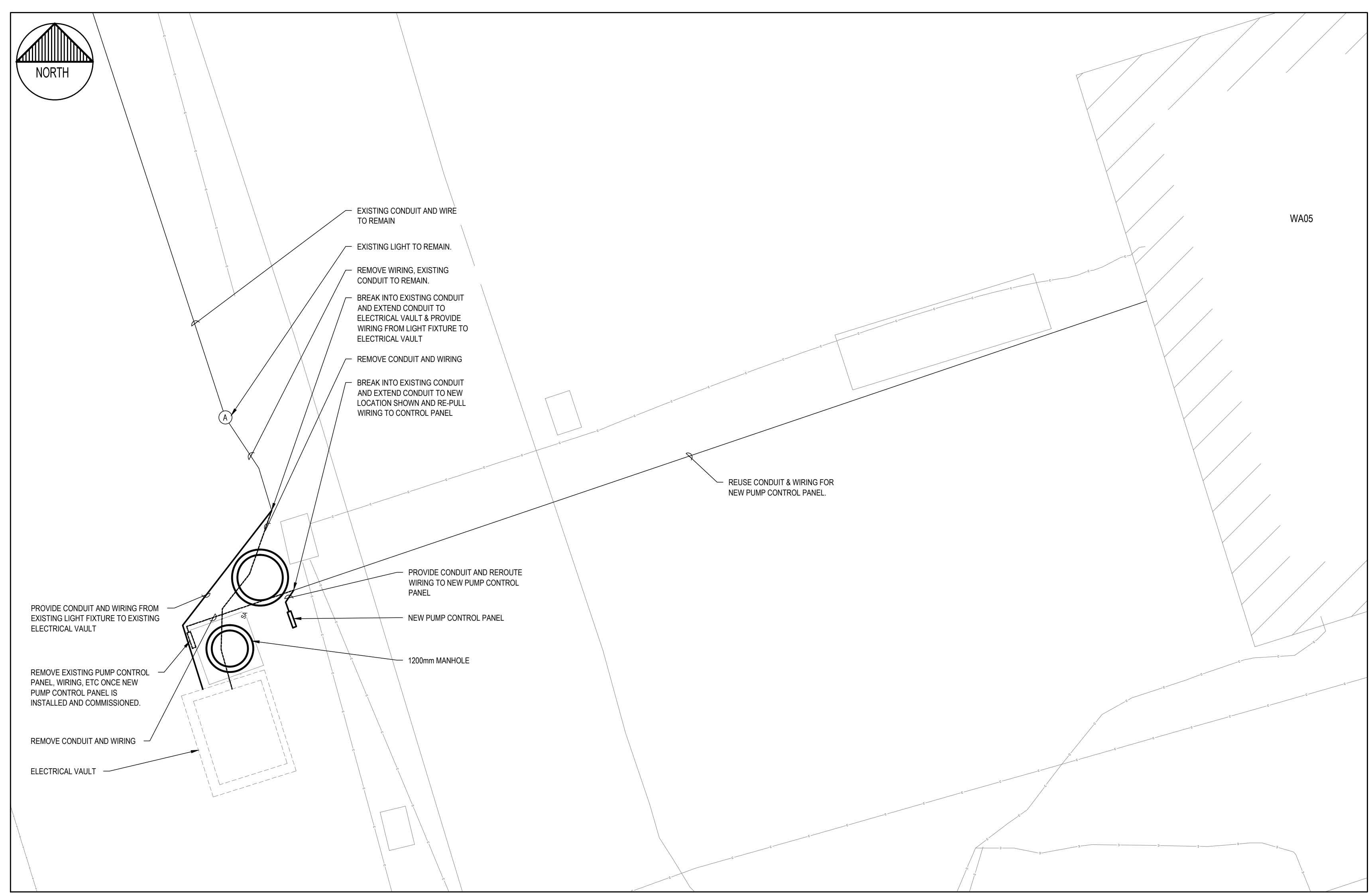
3 SITE PLAN SCALE: 1:100
