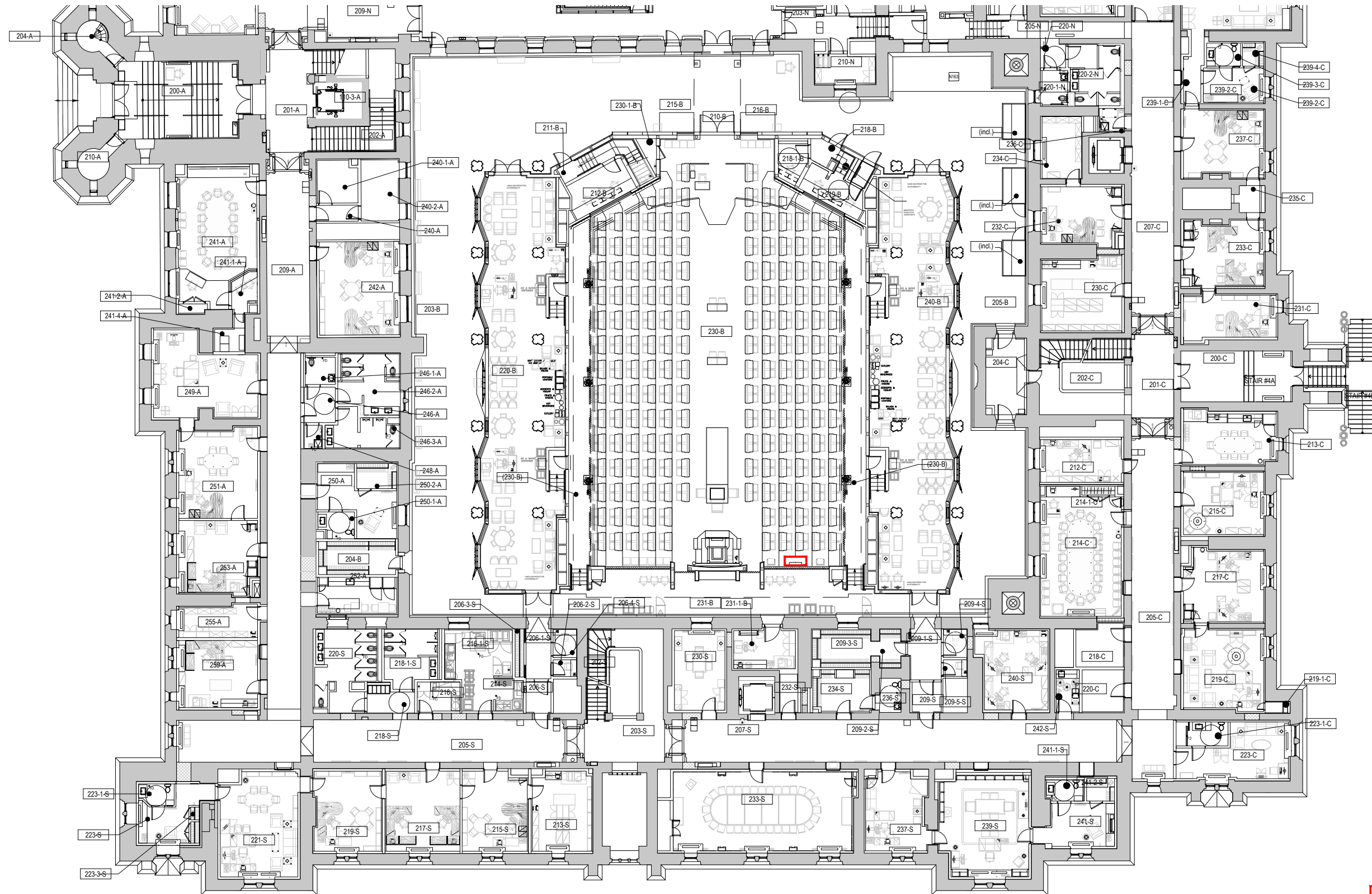
1 01 1:300 LOCATION PLAN - LEVEL 2_SOUTH - SUPERVISOR'S CABINET PLAN DE LOCALISATION DU MEUBLE DU SUPERVISEUR - NIVEAU 2_SUD
