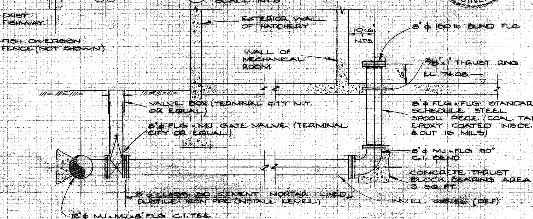
SECTION 2 STATION 0+57.08 SCALE: N.T.S.
