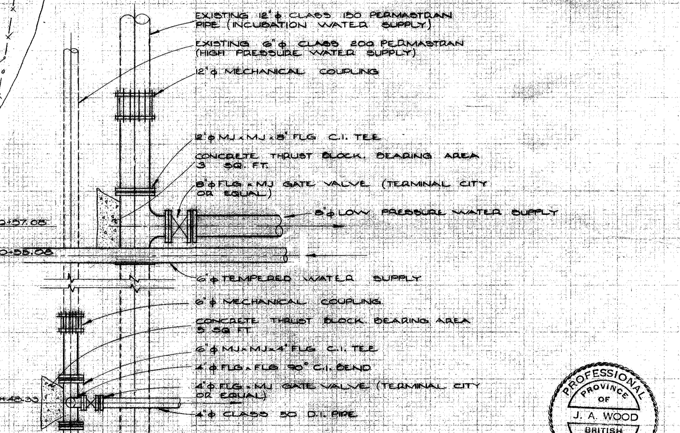
DETAIL A WATER SUPPLY SCALE: N.T.S.
