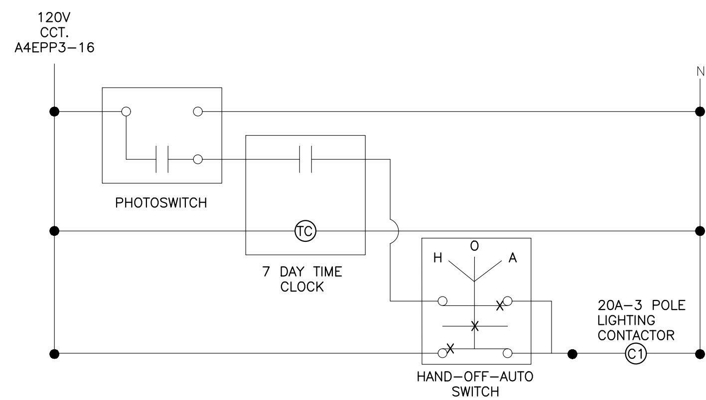
3 EXTERIOR LIGHTING CONTROL DETAILS SCALE: N.T.S.
