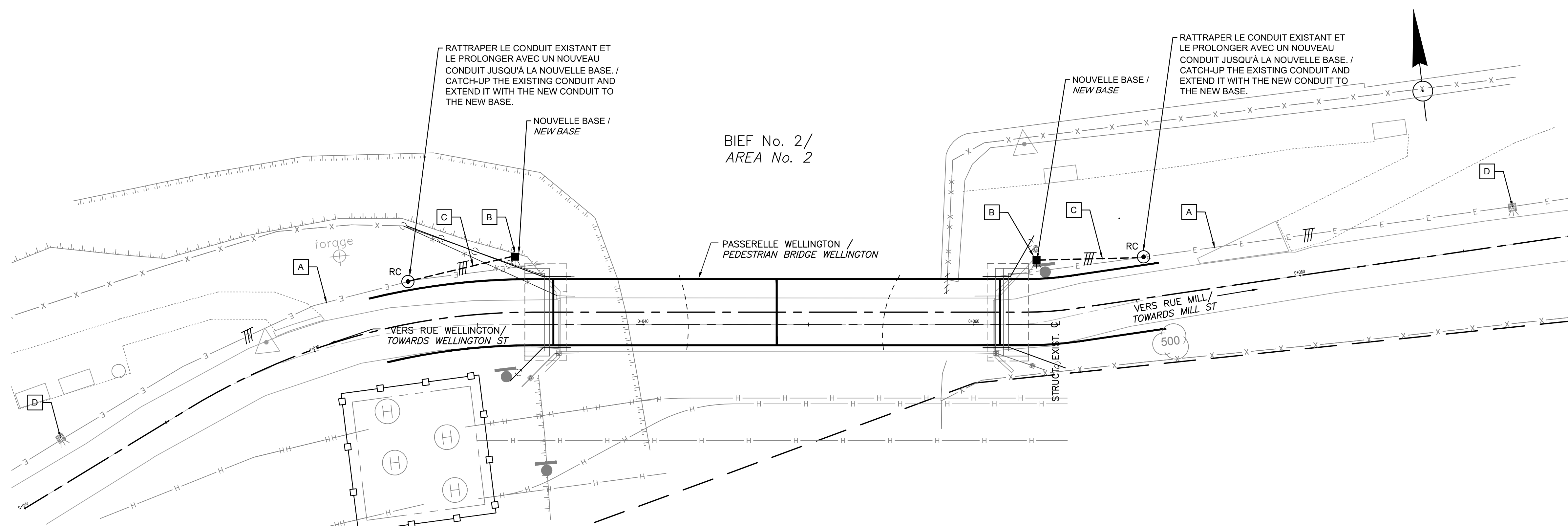
VUE EN PLAN PLAN VIEW ÉCH./SCALE : 1:150
