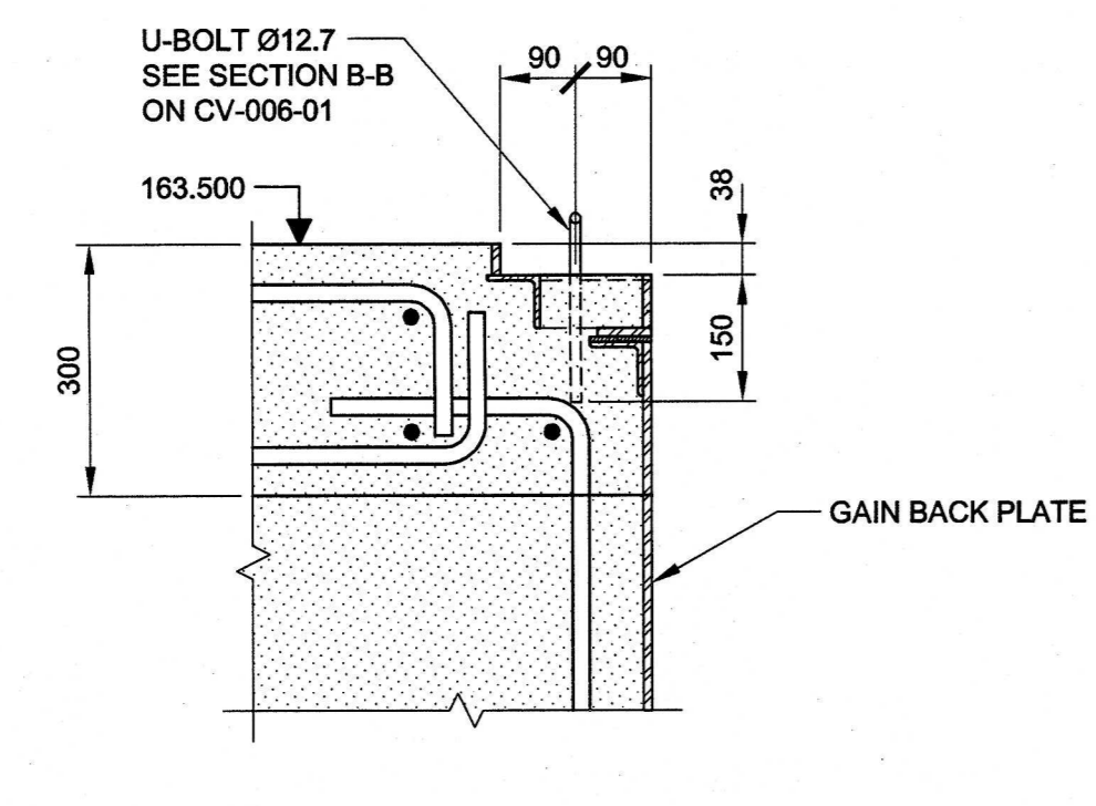
SECTION A-A 1:10
