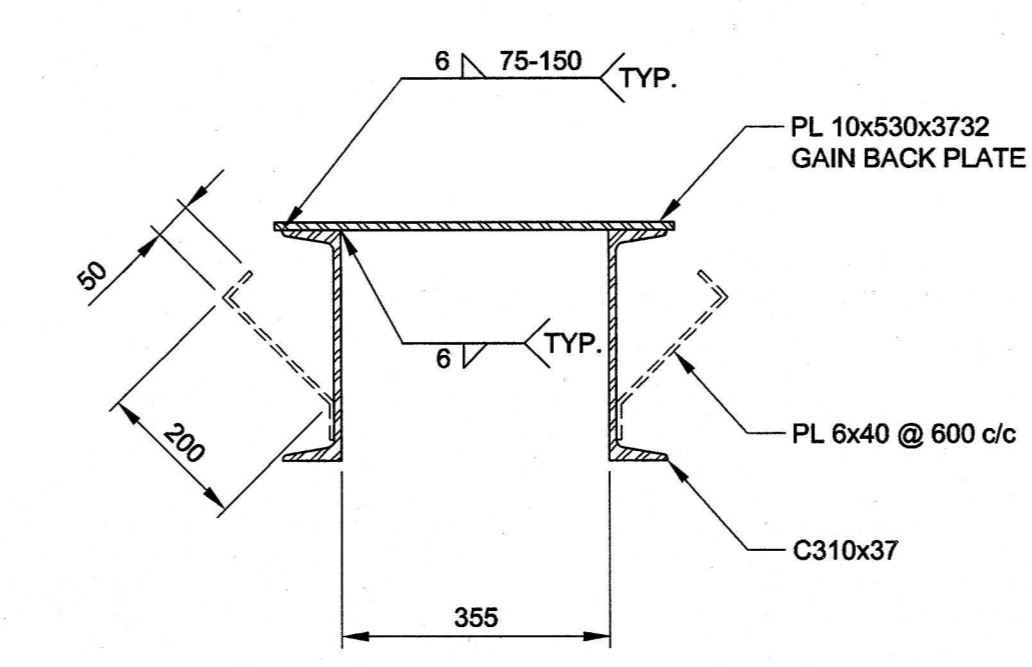
SECTION D-D 1:10
