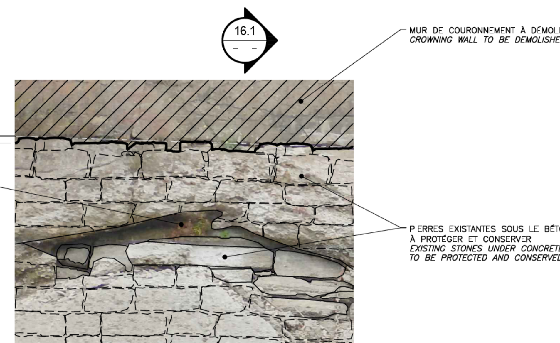
ÉLEVATION / ELEVATION 16.2 ECH./SCALE 1:25
