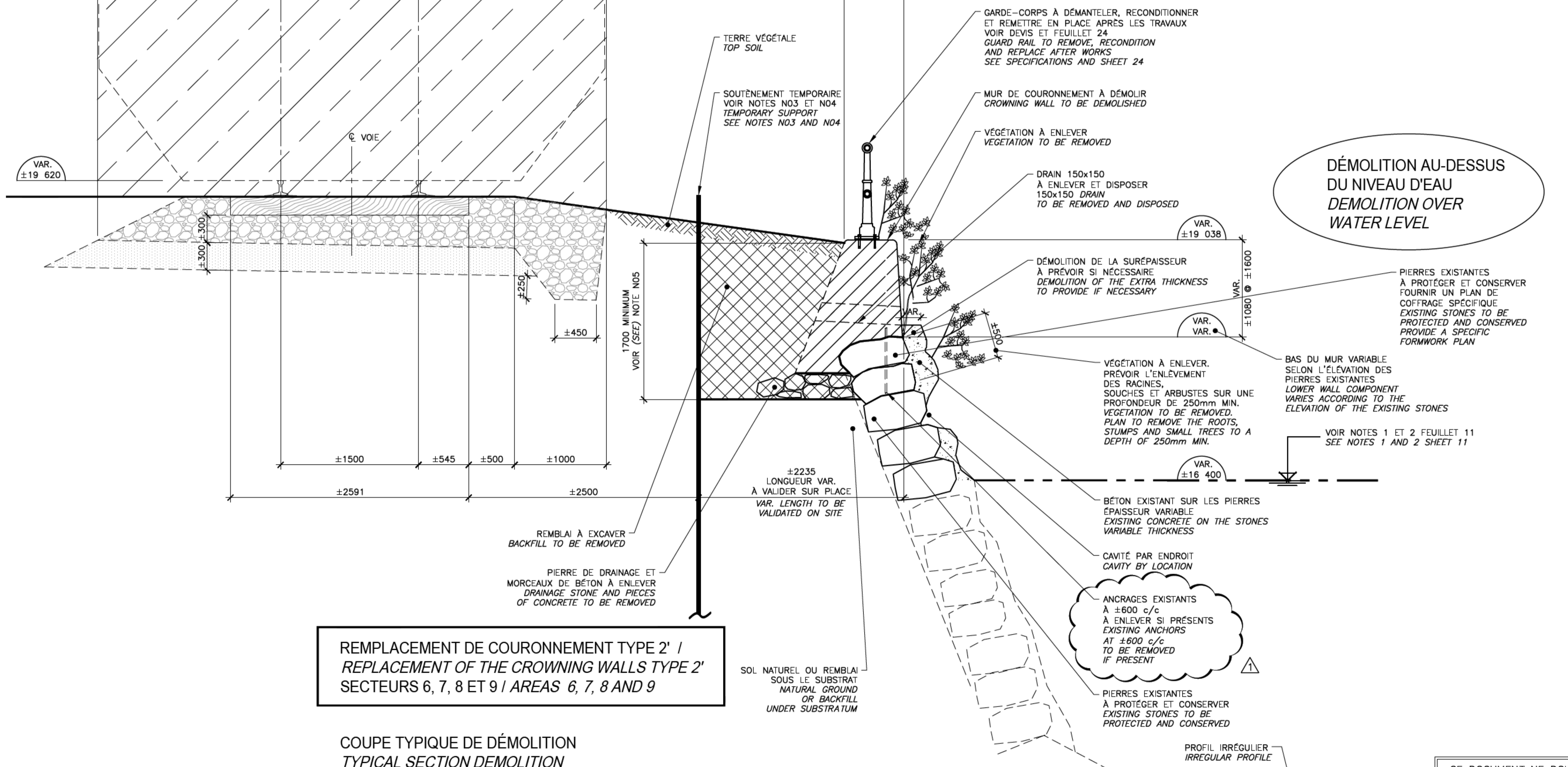
COUPE / SECTION 16.1 ECH./SCALE 1:25
