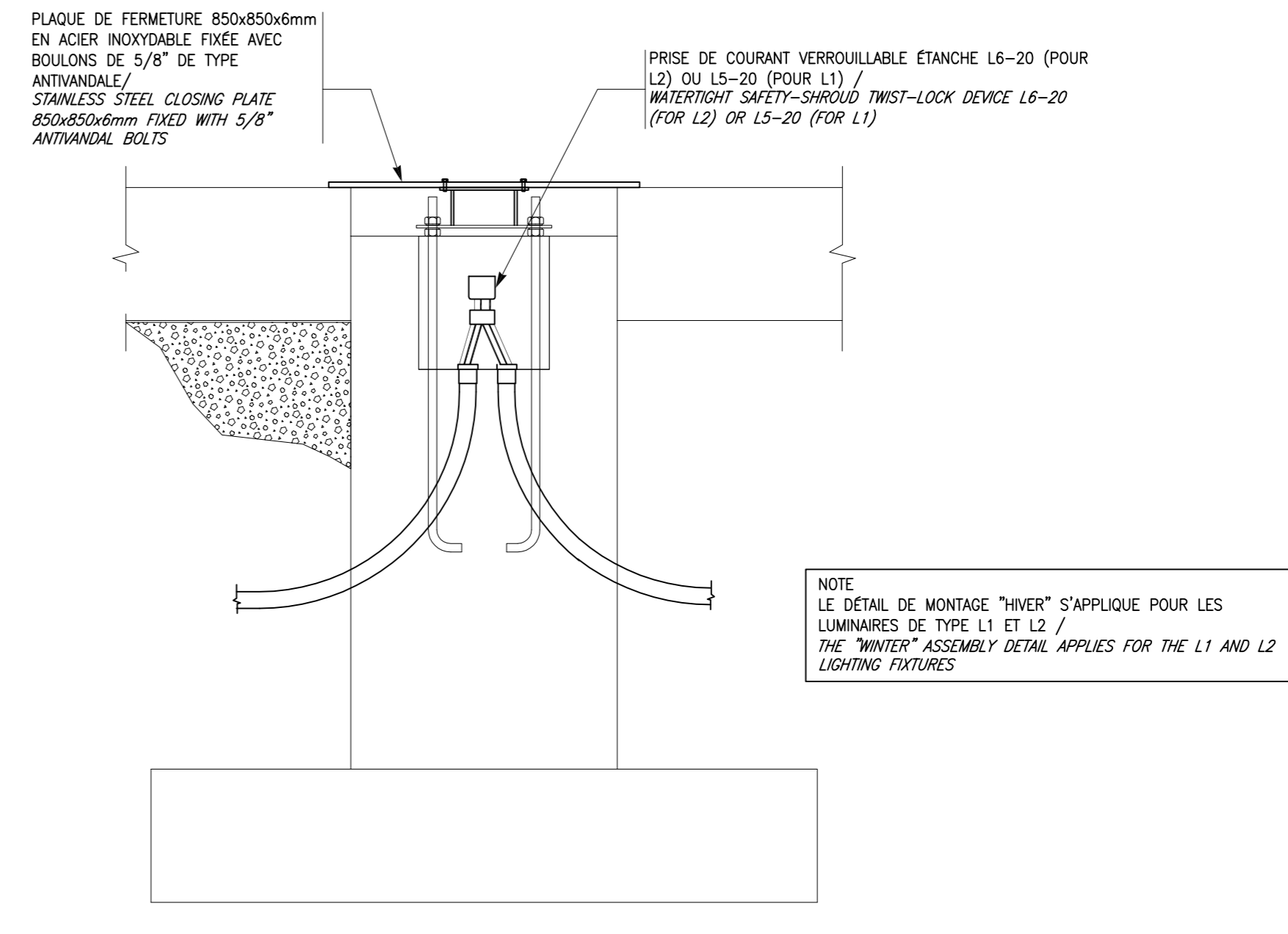
DÉTAIL B: BASE DE BÉTON (MONTAGE "HIVER") / DETAIL B: CONCRETE BASE ("WINTER" ASSEMBLY) ÉCHELLE: AUCUNE / SCALE: NONE
