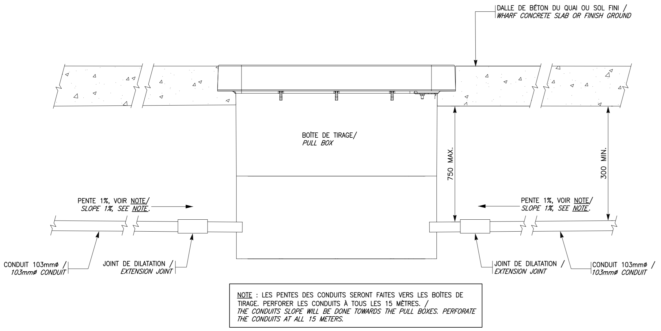
DÉTAIL G: BOÎTE DE TRASSE / DETAIL G: PULL BOX ÉCHELLE: AUCUNE / SCALE: NONE
