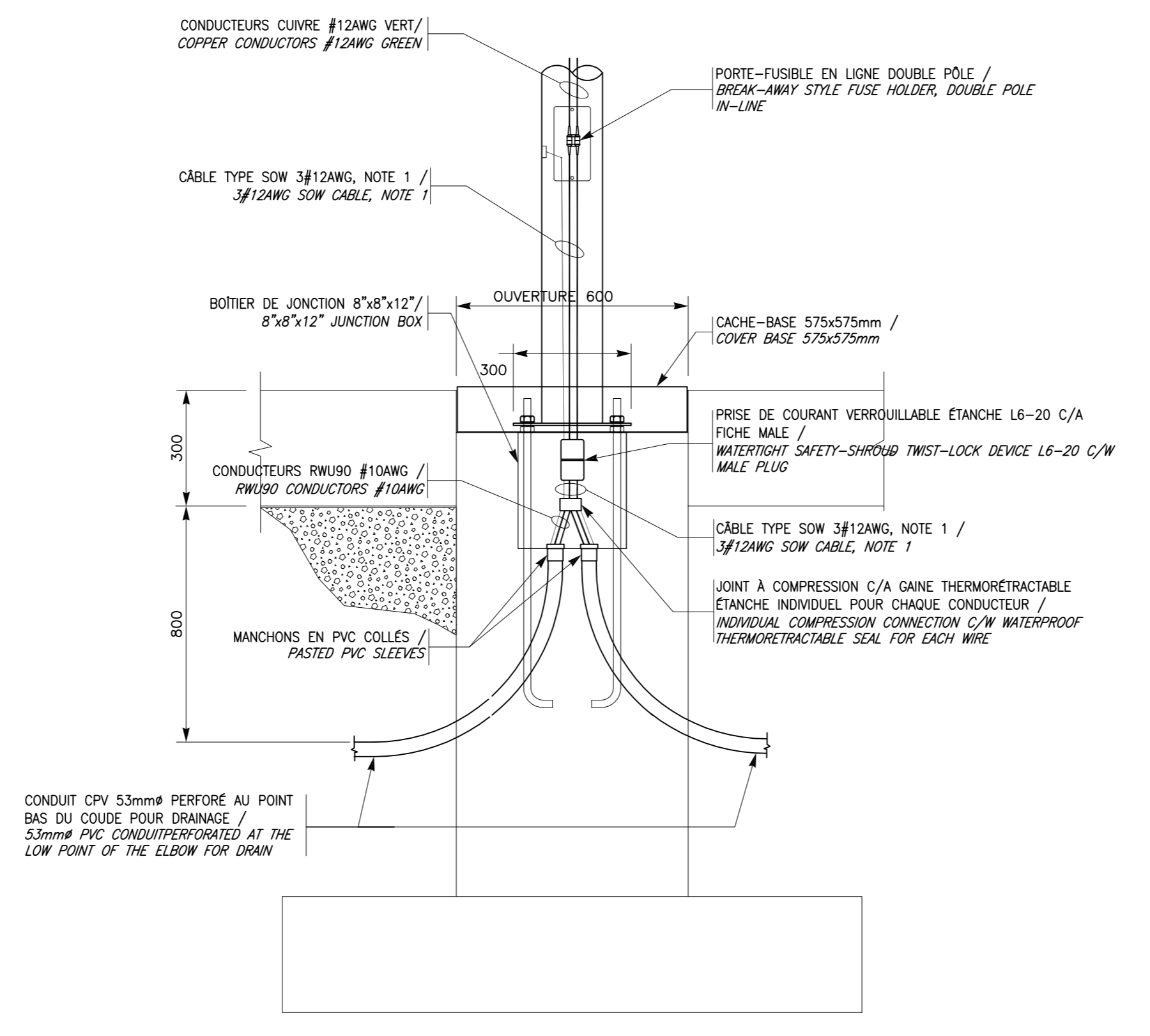
DÉTAIL C: FÛT D'ÉCLAIRAGE TYPE L2 (MONTAGE "ÉTÉ") / DETAIL C: LIGHTING POLE TYPE L2 ("SUMMER" ASSEMBLY) ÉCHELLE: AUCUNE / SCALE: NONE
