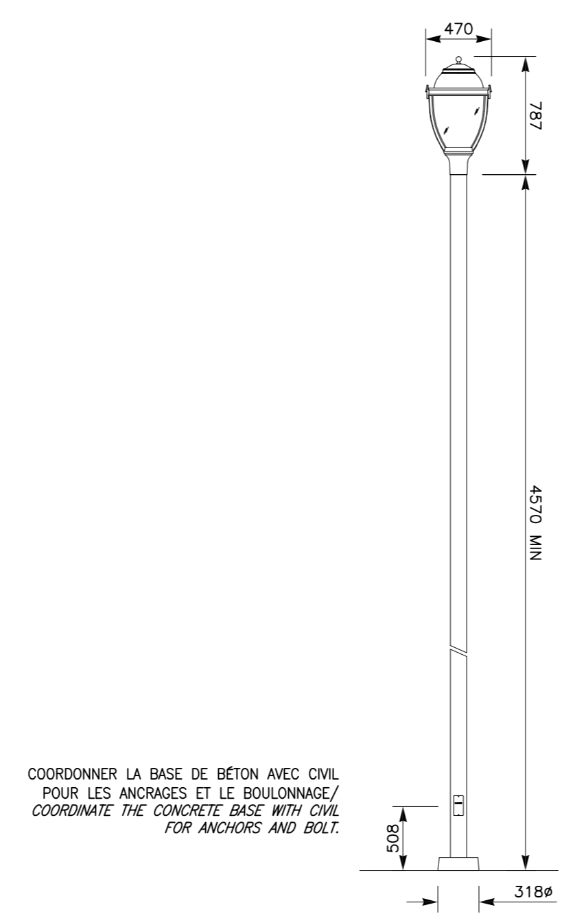
DÉTAIL C: FÛT D'ÉCLAIRAGE TYPE L2 / DETAIL C: LIGHTING POLE TYPE L2 ÉCHELLE: AUCUNE / SCALE: NONE
