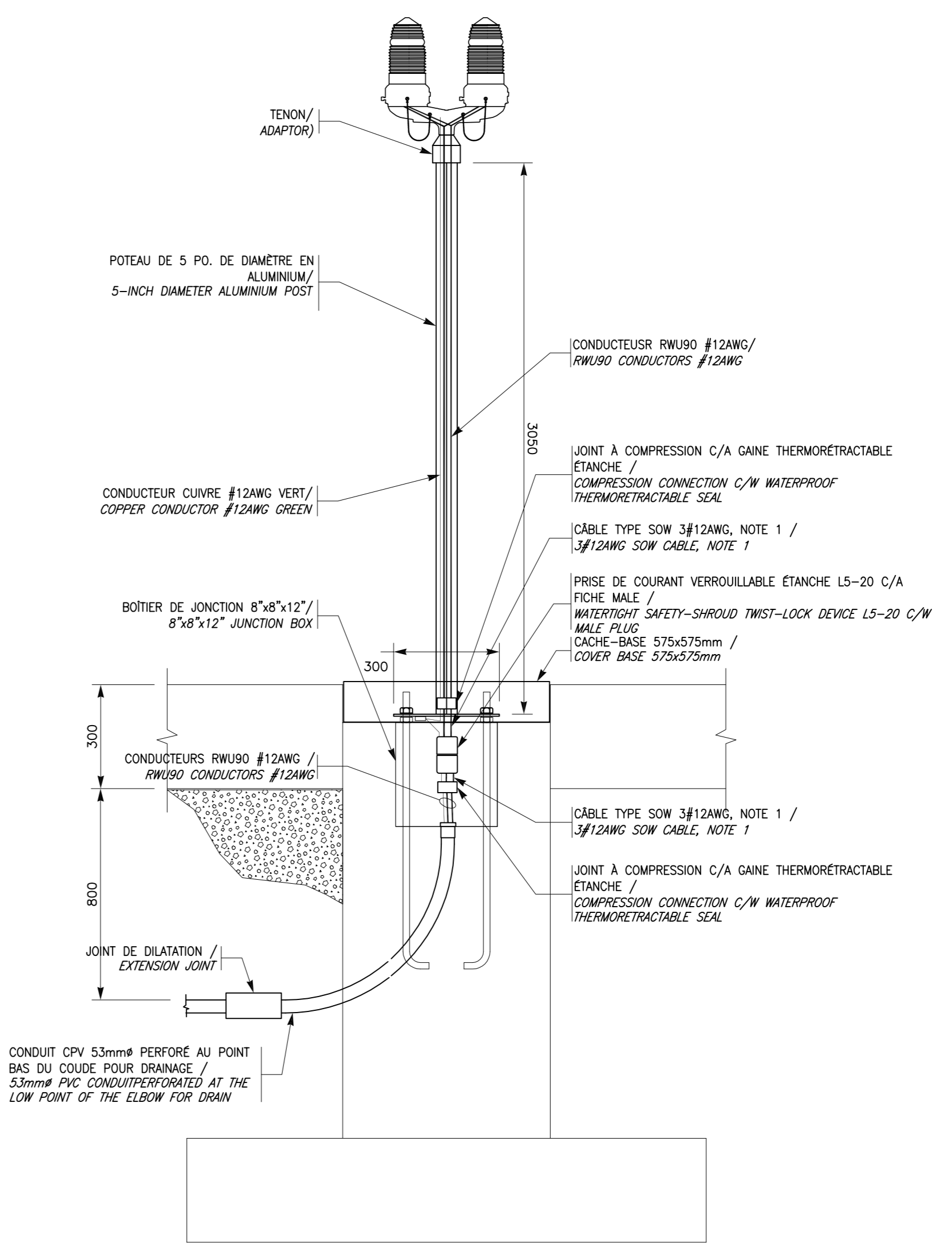
DÉTAIL E: FEU DE NAVIGATION TYPE I1 (MONTAGE "ÉTÉ") / DETAIL E: NAVIGATION LIGHT TYPE I1 ("SUMMER" ASSEMBLY) ÉCHELLE: AUCUNE / SCALE: NONE
