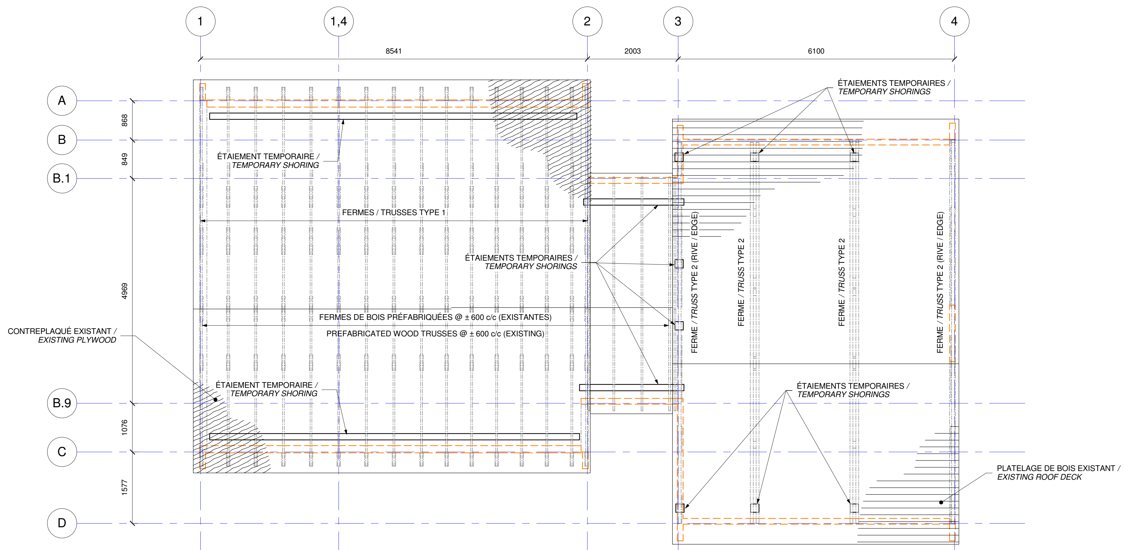
VUE EN PLAN DÉMOLITION ET ÉTAIEMENT TEMPORAIRE - TOITURE / DEMOLITION AND TEMPORARY SHORING PLAN VIEW - ROOF
