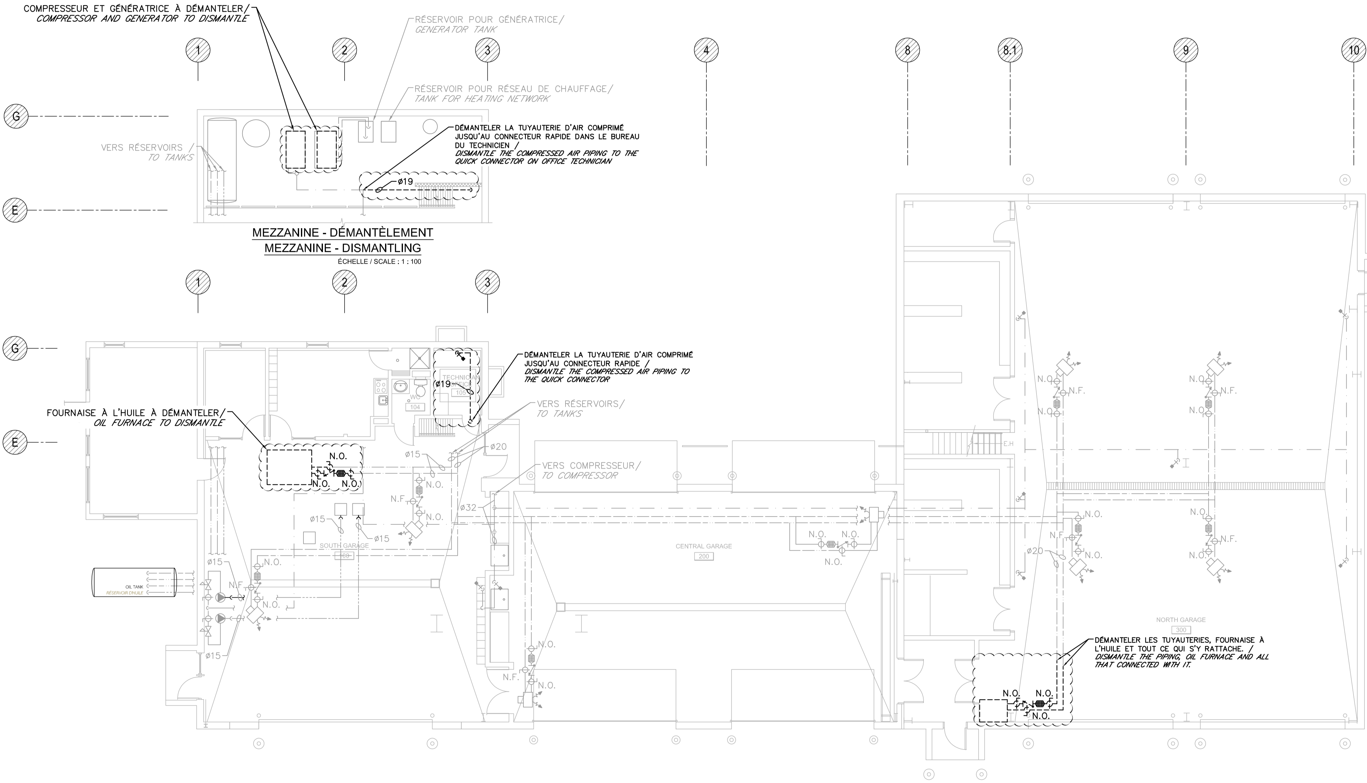
REZ-DE-CHAUSSÉE - DÉMANTÈLEMENT GROUND FLOOR - DISMANTLING ÉCHELLE / SCALE: 1:100
