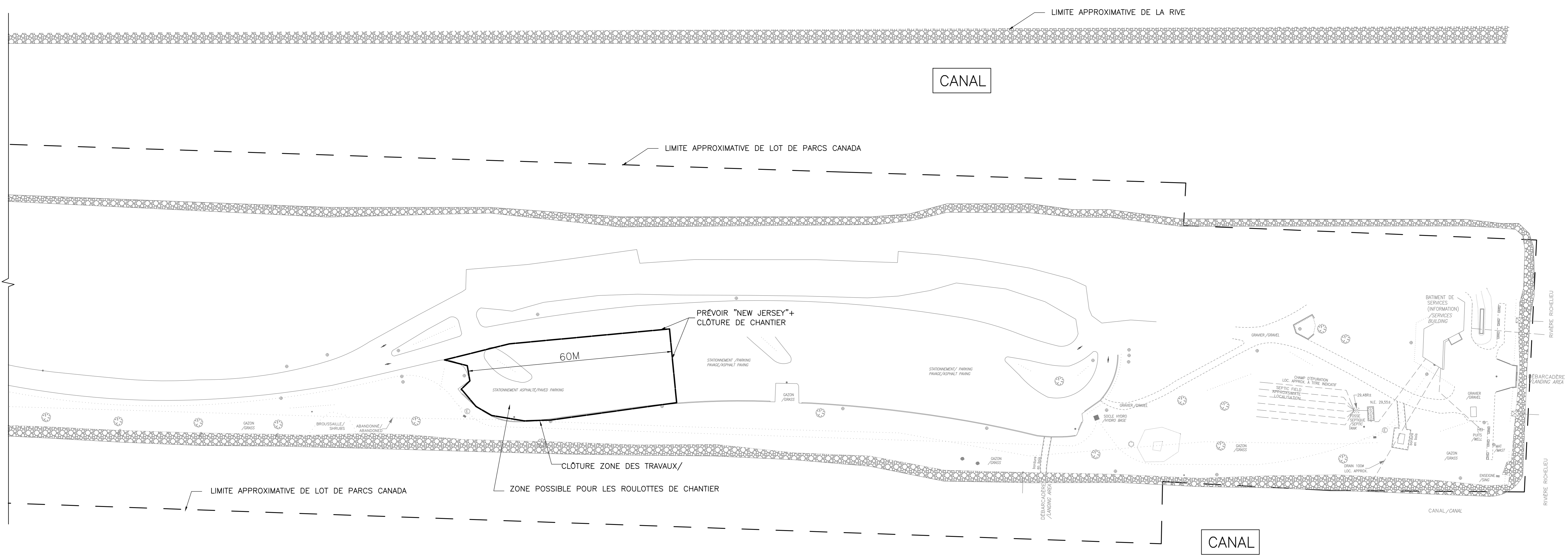
VUE EN PLAN INSTALLATION DE CHANTIER (QUAI ET RAMPE DE LA 61ième AVENUE)
