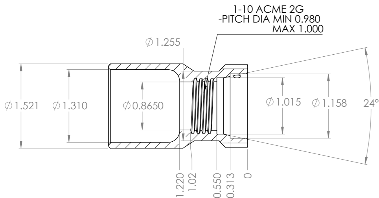
SECTION A-A
