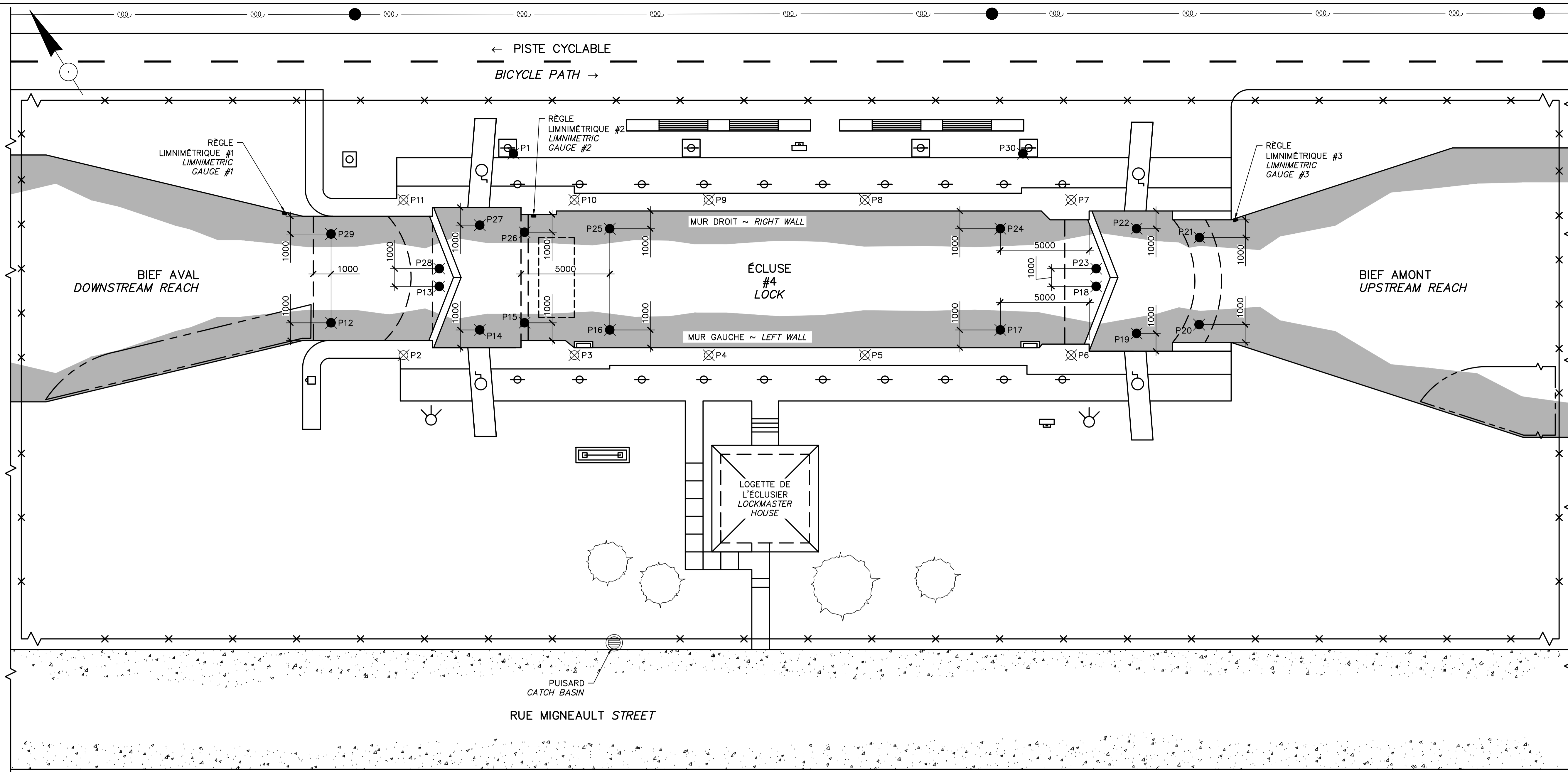
VUE EN PLAN 18.1 PLAN D'ENSEMBLE PLAN VIEW GENERAL LAYOUT ÉCH. ~ SCALE 1:125
