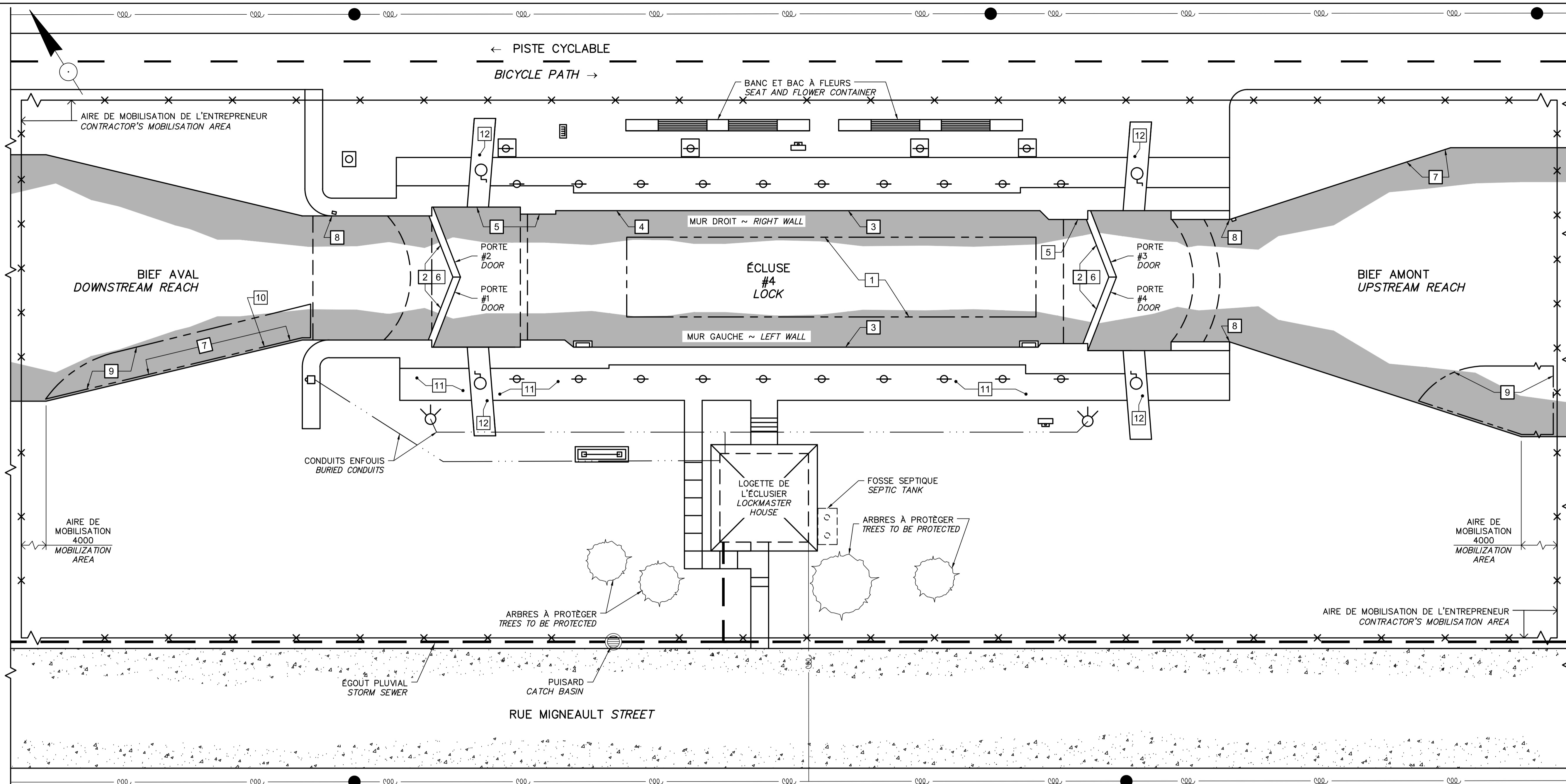
VUE EN PLAN 3.1 PLAN D'ENSEMBLE PLAN VIEW GENERAL LAYOUT ÉCH. ~ SCALE 1:125
