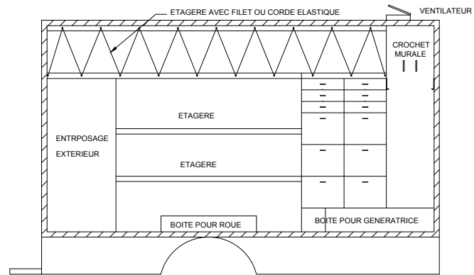
ELEVATION : E1
