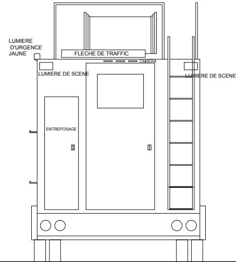
ELEVATION : E5
