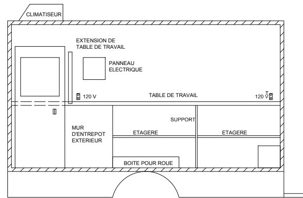
ELEVATION : E2
