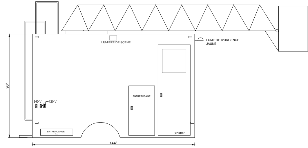
ELEVATION : E3
