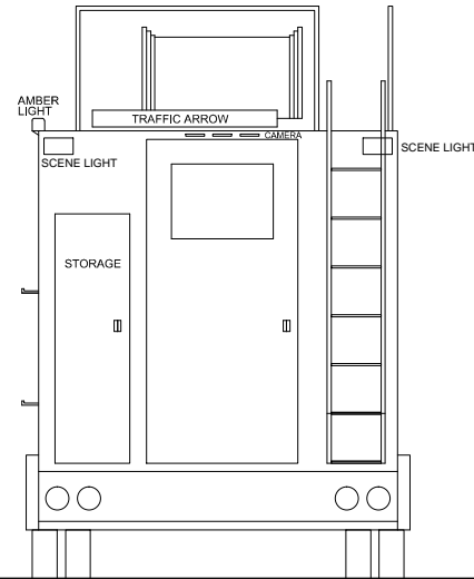
ELEVATION : E5
