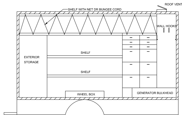
ELEVATION : E1
