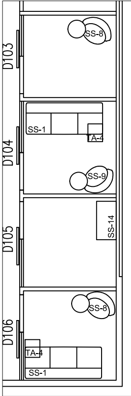
PLAN DU MOBILIER - CB-G
