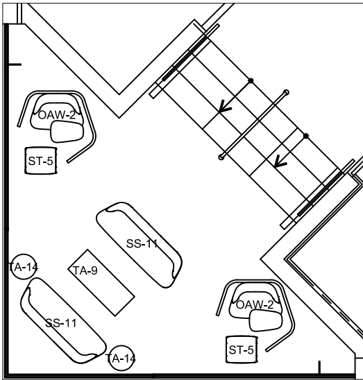
PLAN DU MOBILIER - CB-I ÉCHELLE: 1/8"=1'-0"
