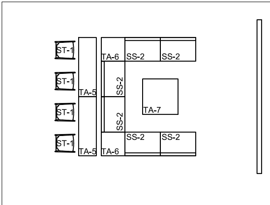
FURNITURE LAYOUT - CB-A SCALE: 1/8"=1'-0"
