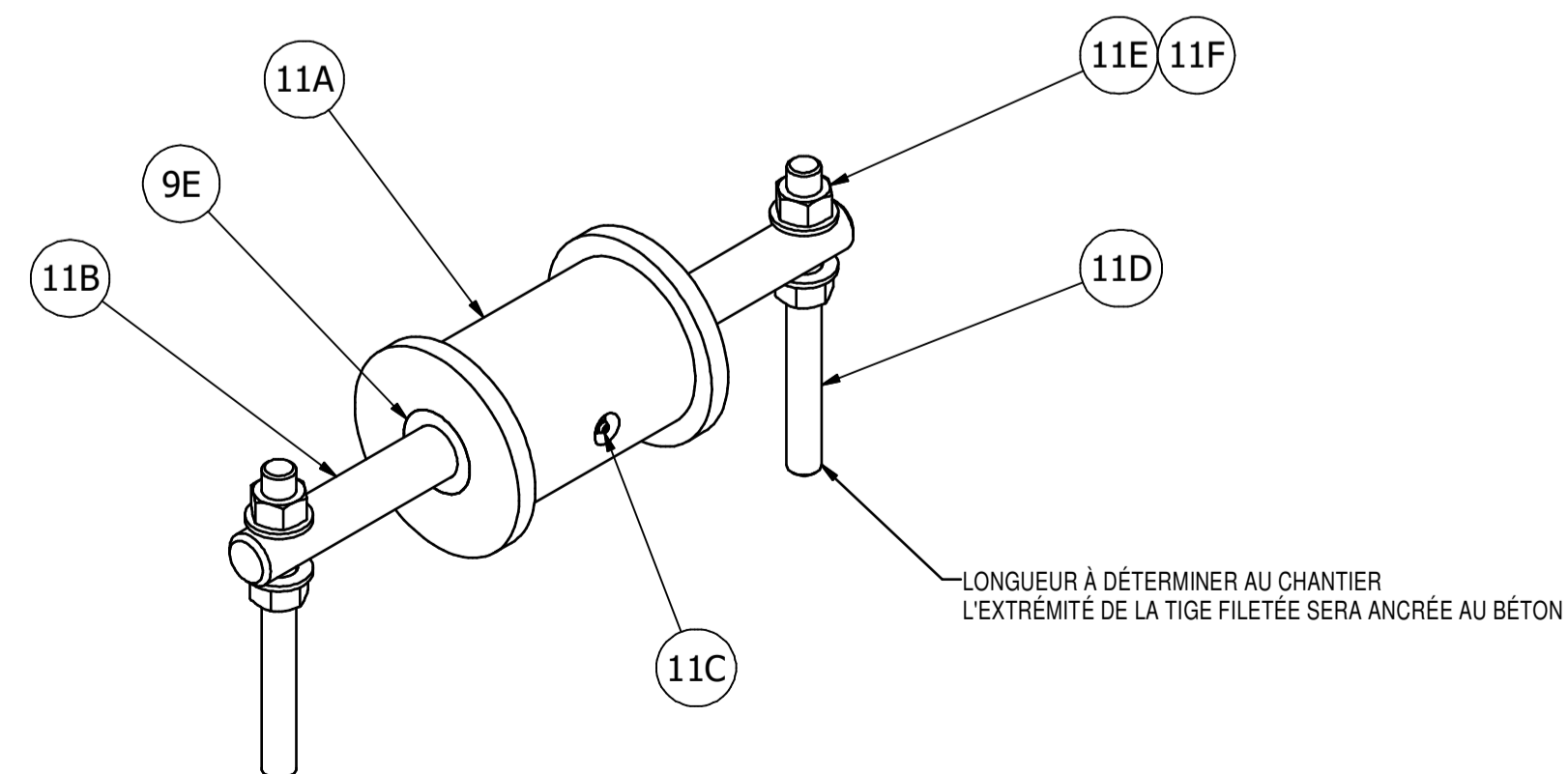
ROULEAU DE GUIDAGE 11 VUE ISOMÉTRIQUE GUIDING ROLLER 15 17 ISOMETRIC VIEW N.À.É. ~ N.T.S.
