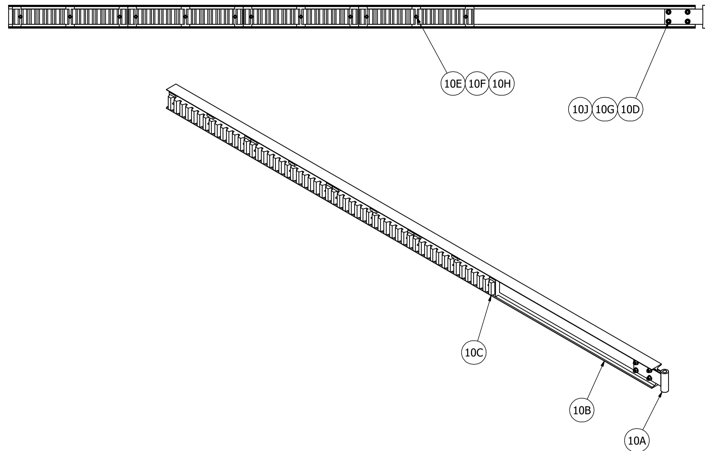
ASSEMBLAGE DE LA CRÉMAILLÈRE 10 VUE ISOMÉTRIQUE RACK ASSEMBLY 15 17 ISOMETRIC VIEW N.À.É. ~ N.T.S.
