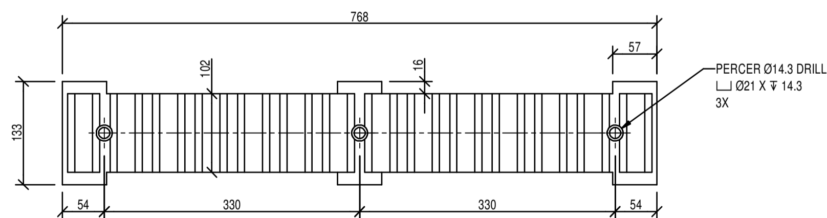
ÉLÉVATION - ELEVATION
