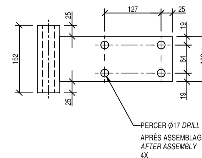
ÉLÉVATION - ELEVATION
