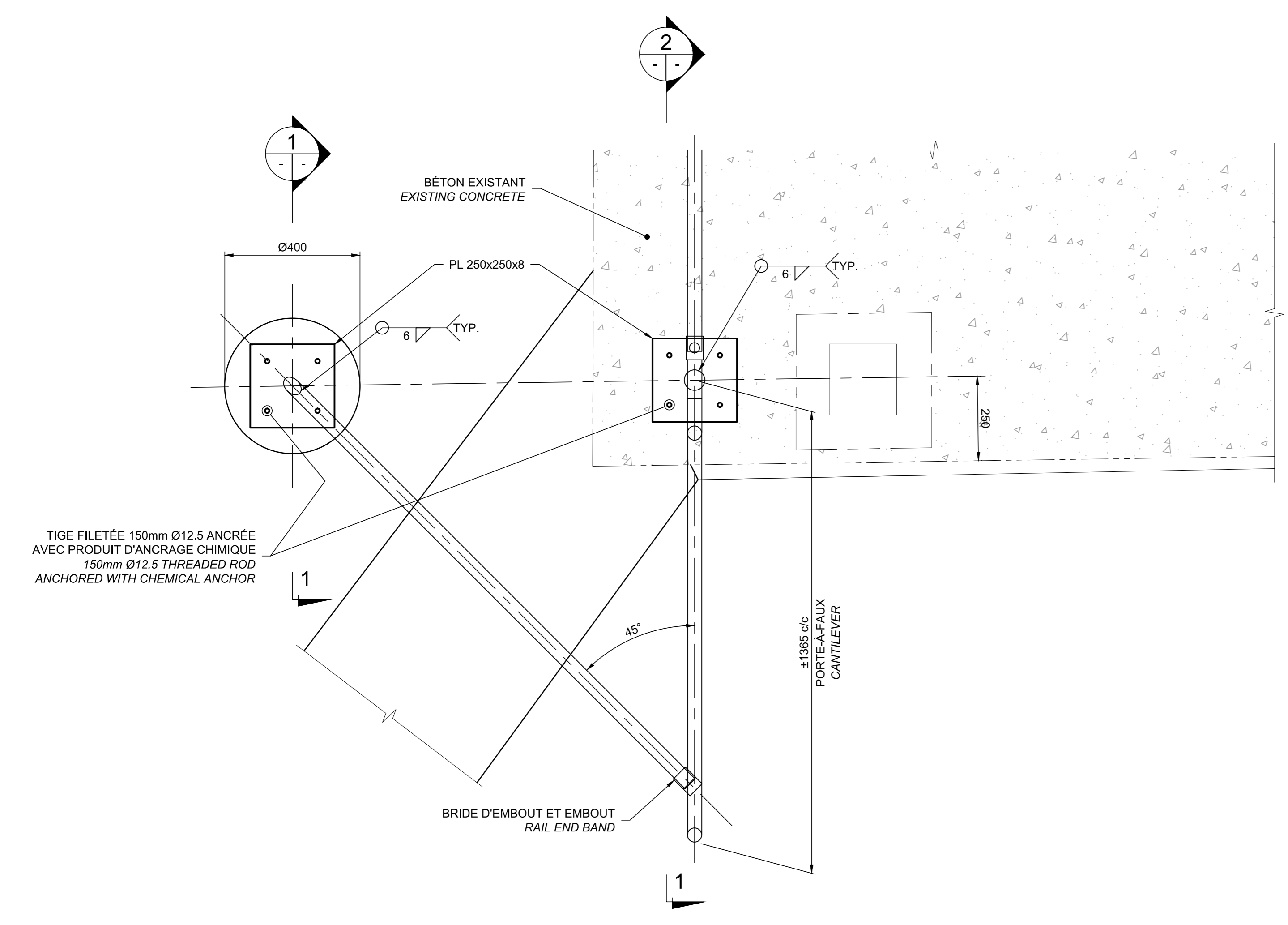
DÉTAIL / DETAIL A NON À L'ÉCHELLE / NOT TO SCALE
