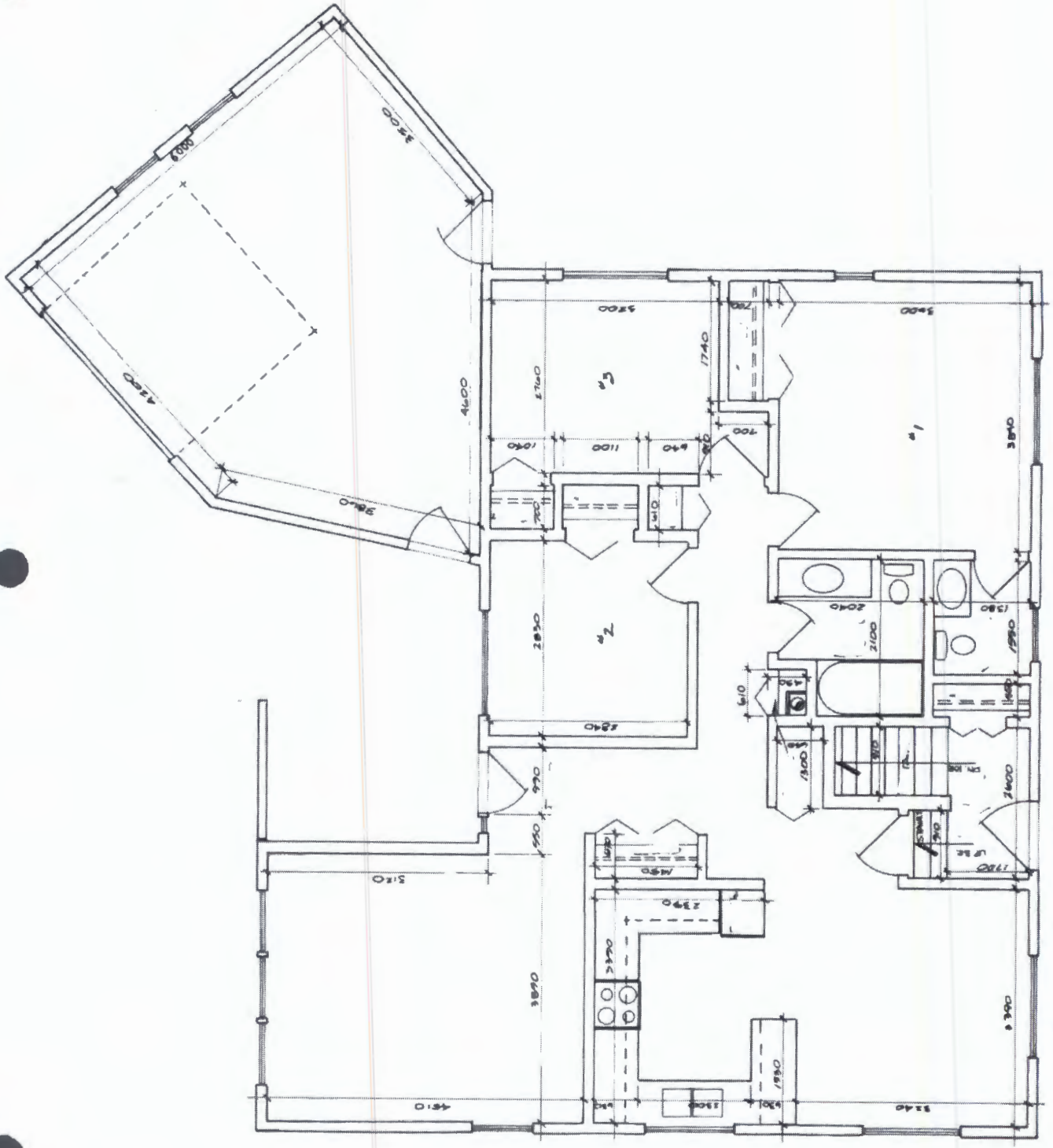
SWAN HILLS, ALBERTA MAIN FLOOR PLAN SCALE: N.T.S. 84 NOV 08
