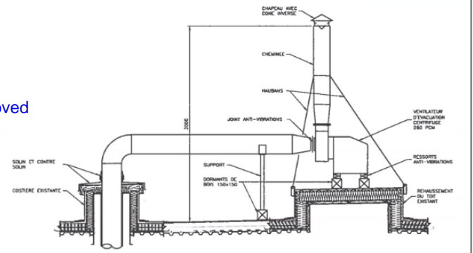
DETAIL TYPE - VENTILATEUR D'EVACUATION AU TOIT ECHELLE: AUCUNE
