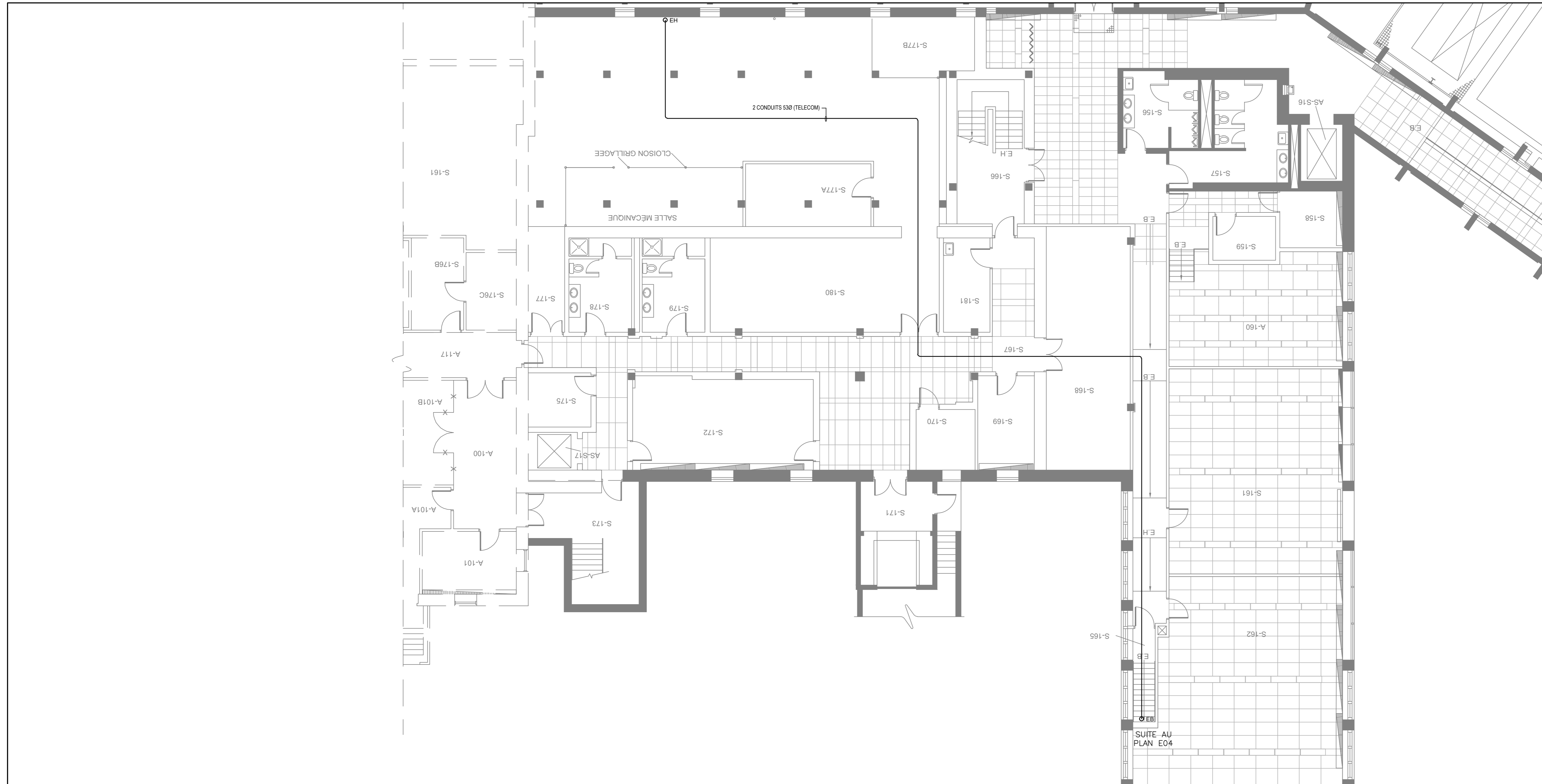
BLOCS C/N - 1er ÉTAGE BLOCS C/N - 1st FLOOR
