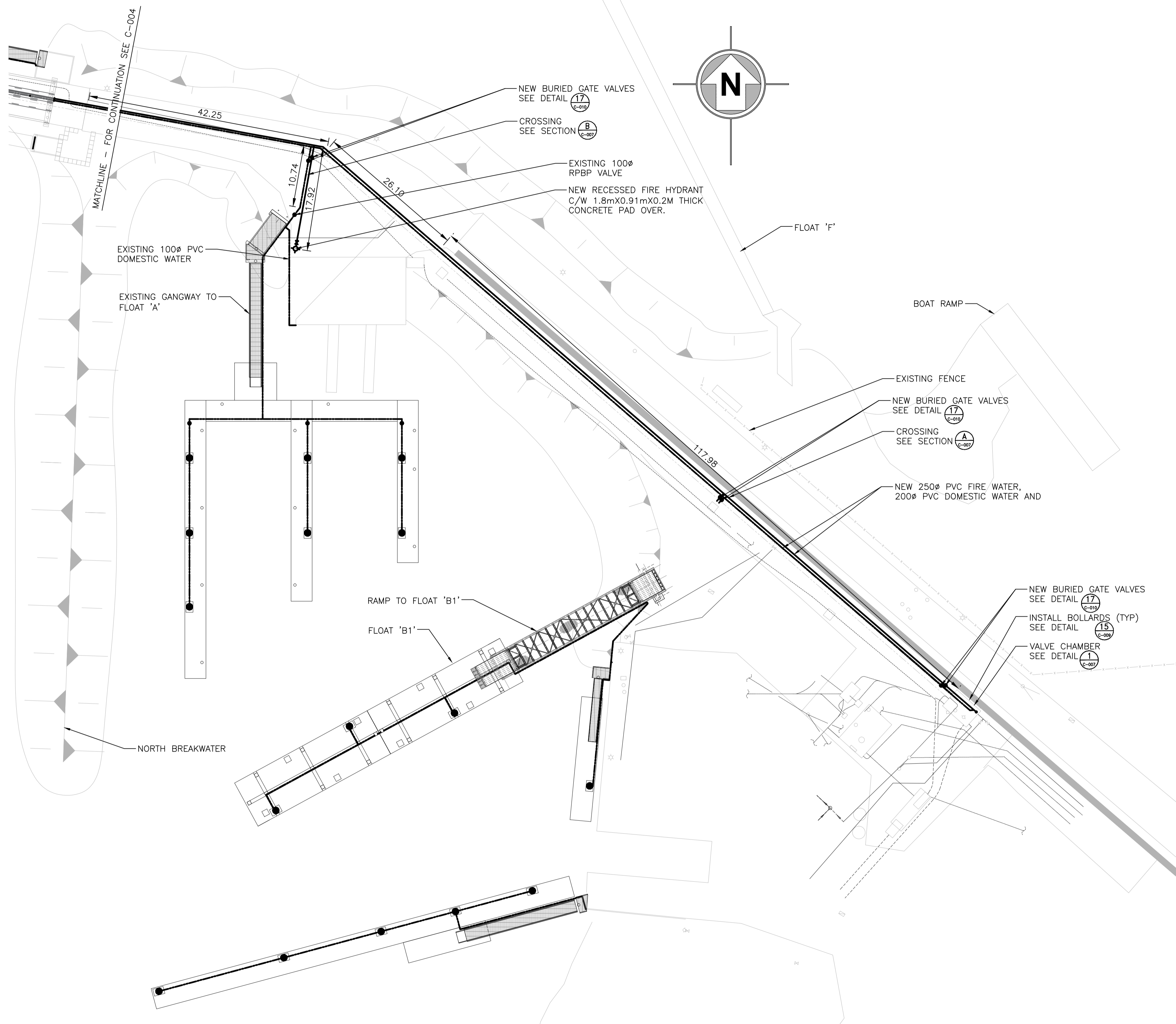
PLAN - CAUSEWAY SCALE: 1:400
