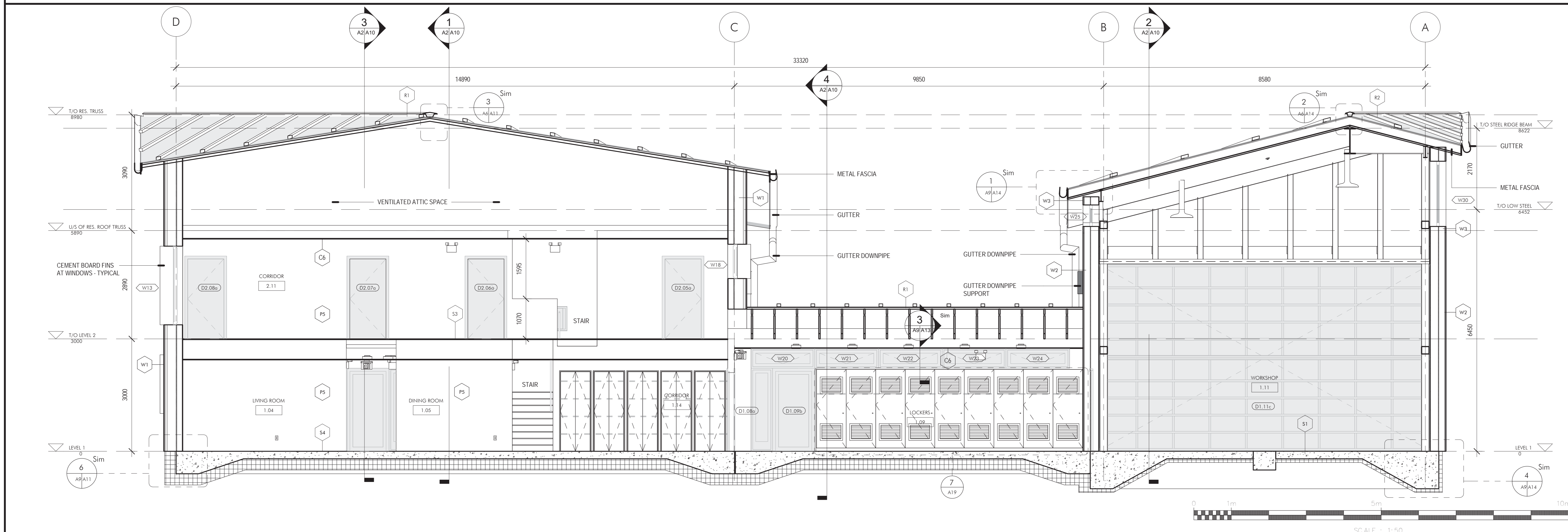
2 Section BB A9 A2
