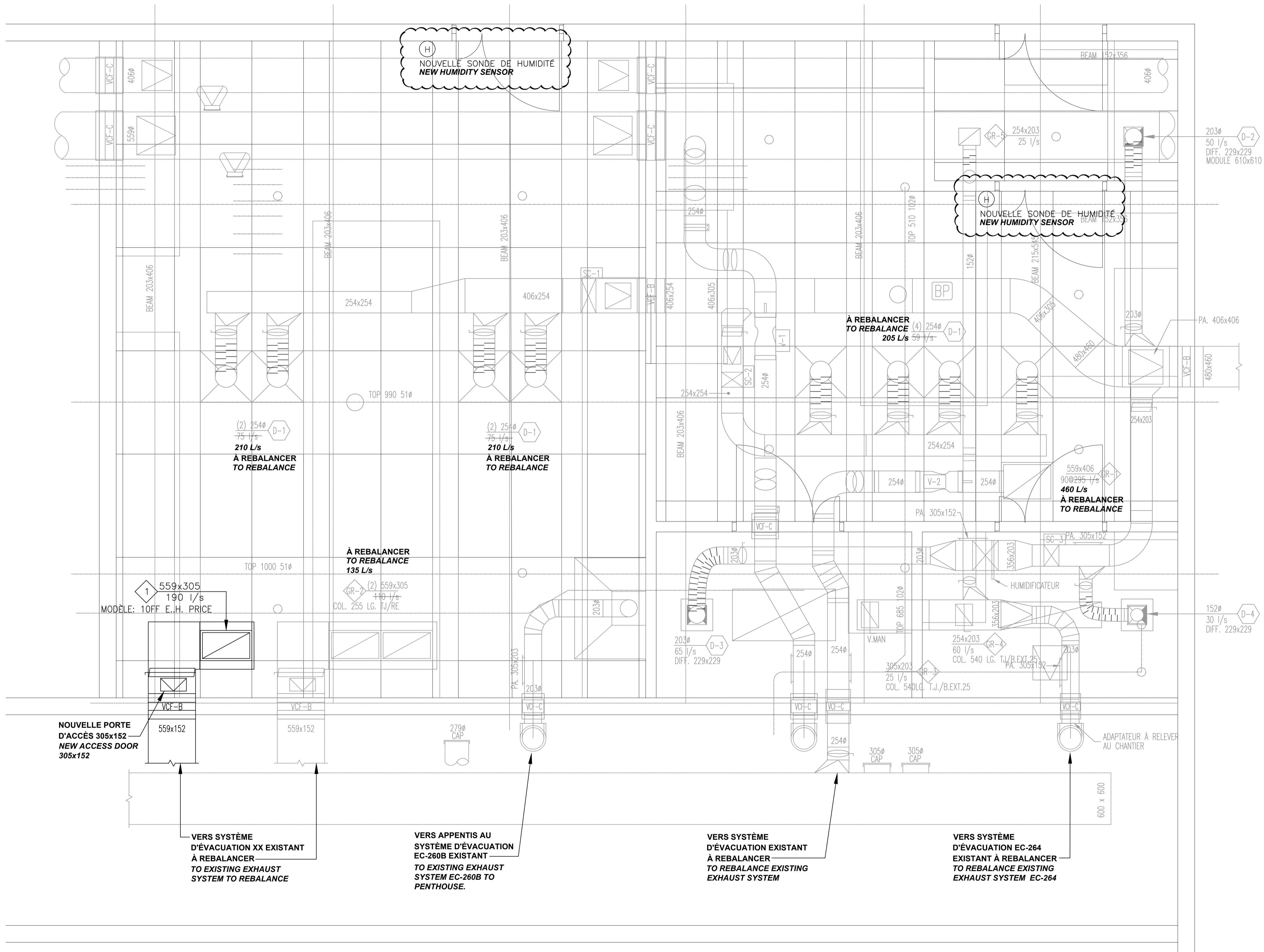
1 M-05 VENTILATION - 2e ÉTAGE - CONSTRUCTION VENTILATION - SECOND FLOOR - NEW ÉCHELLE: 1:50 SCALE: 1:50
