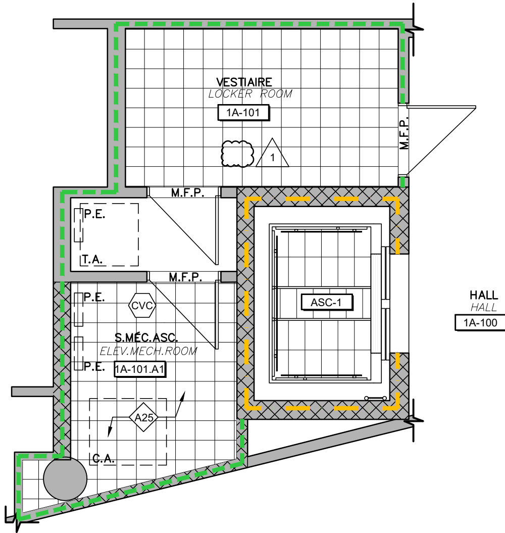
1 13 13 PLAN ASCENSEUR NO.1 ET S.MÉC.ASC – CONSTRUCTION PLAN ELEVATOR NO.1 AND ELEV.MECH.ROOM – CONSTRUCTION
