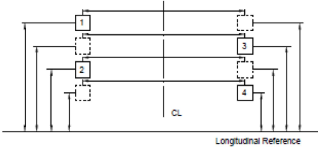
Référence longitudinale
