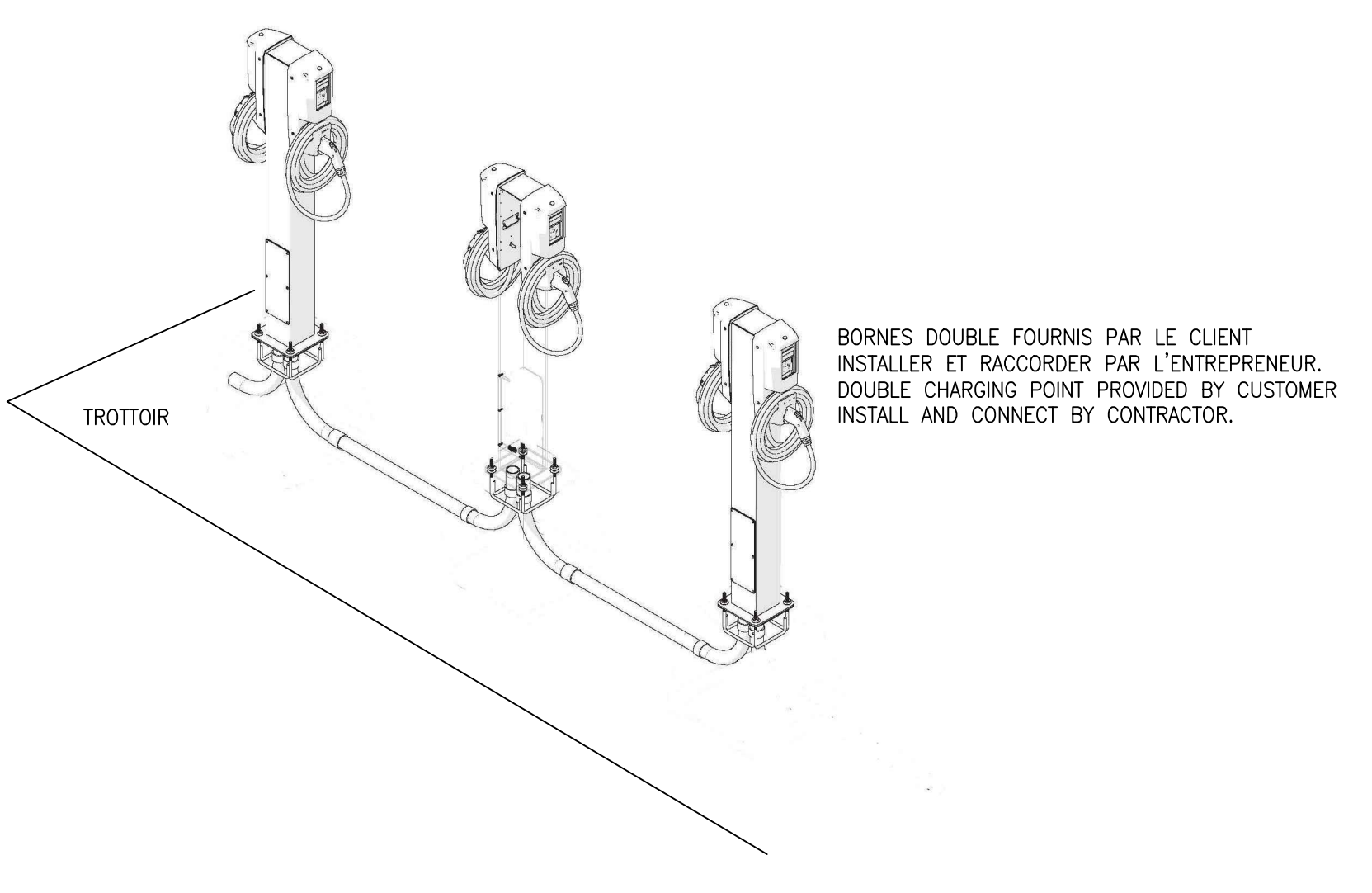
02 - INSTALLATION TYPE DE TROIS BORNES ÉLECTRIQUE TYPICAL INSTALLATION OF THREE CHARGING POINT ÉCHELLE / SCALE : AUCUNE / NONE
