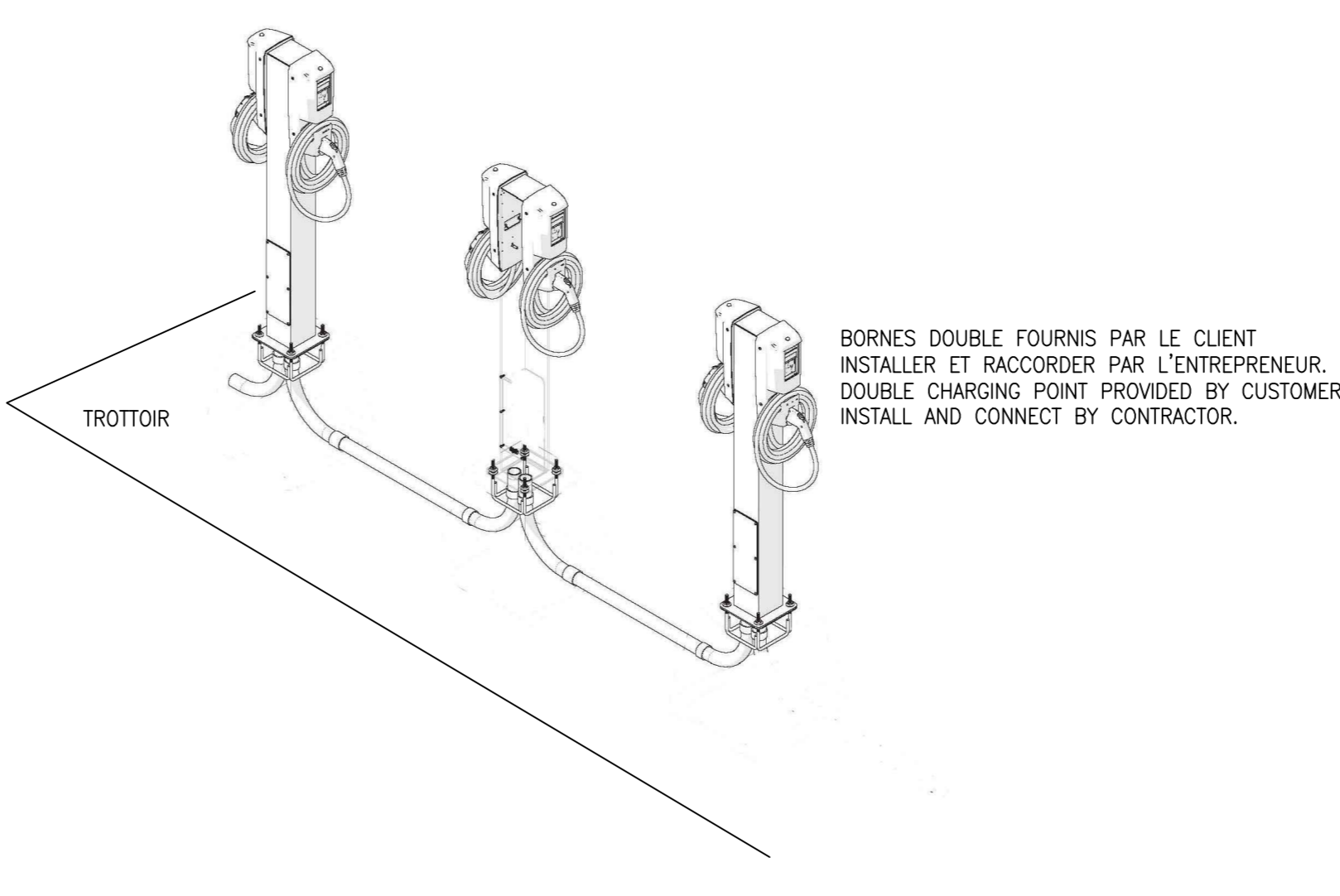
02 - INSTALLATION TYPE DE TROIS BORNES ÉLECTRIQUE TYPICAL INSTALLATION OF THREE CHARGING POINT ÉCHELLE / SCALE : AUCUNE / NONE
