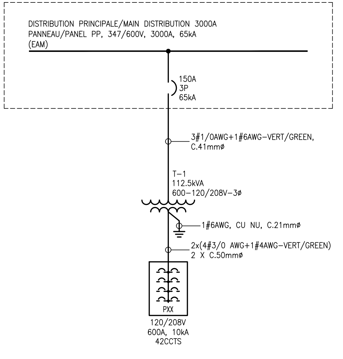
01 - SCHÉMA UNIFILAIRE SINGLE LINE DIAGRAM ÉCHELLE / SCALE : AUCUNE / NONE
