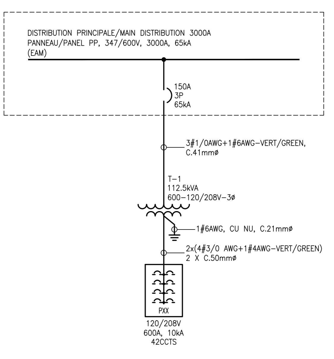
SCHÉMA UNIFILAIRE SINGLE LINE DIAGRAM ÉCHELLE / SCALE : AUCUNE / NONE
