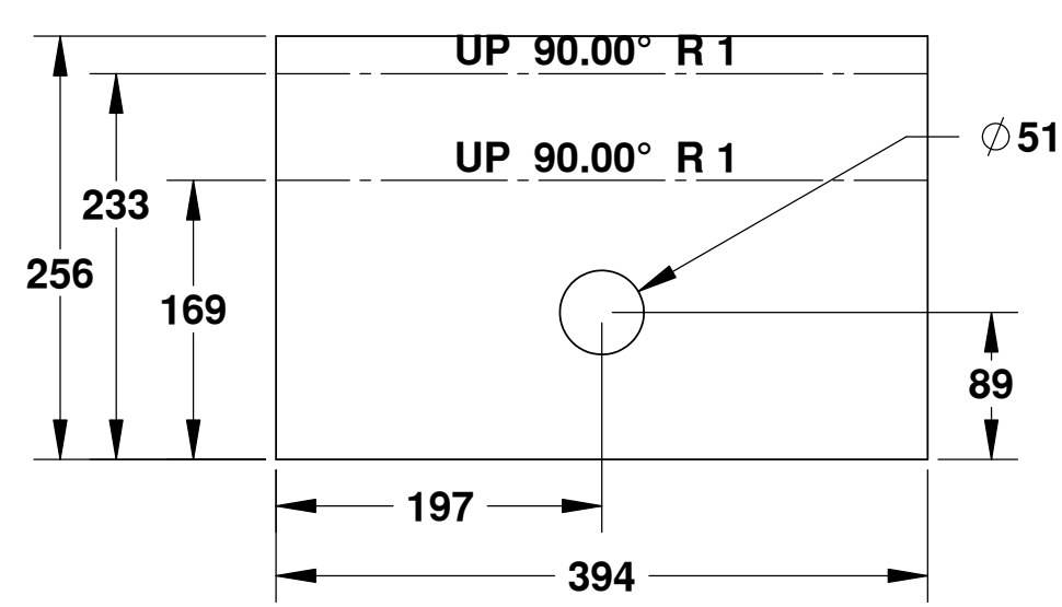
MOUNTING PLATE SCALE: 1-5
