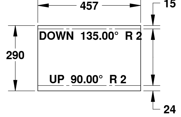
DIVIDER PLATE SCALE: 1-10
