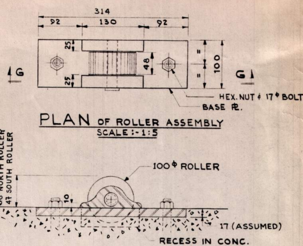
SECTION G-G SCALE: 1:5
