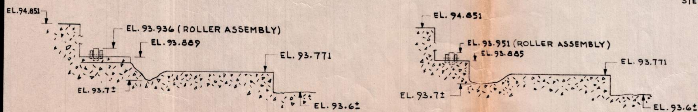
SECTION D-D SCALE: 1:20
