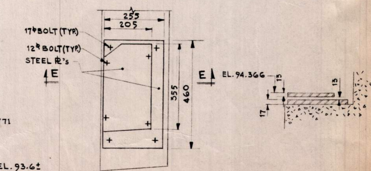
DETAIL-1 SCALE: 1:10
