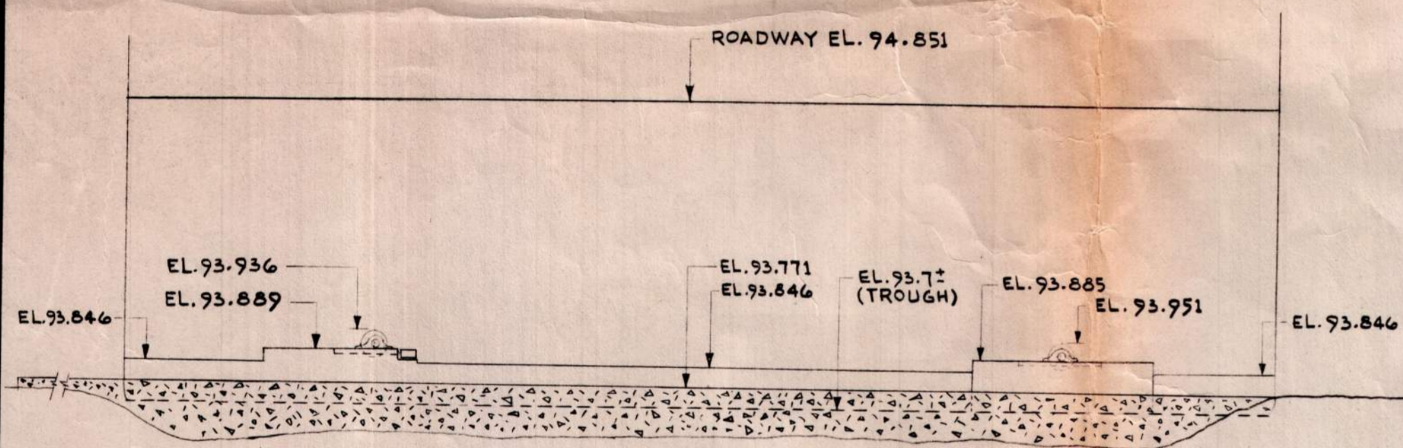
ELEVATION A-A SCALE: 1:20
