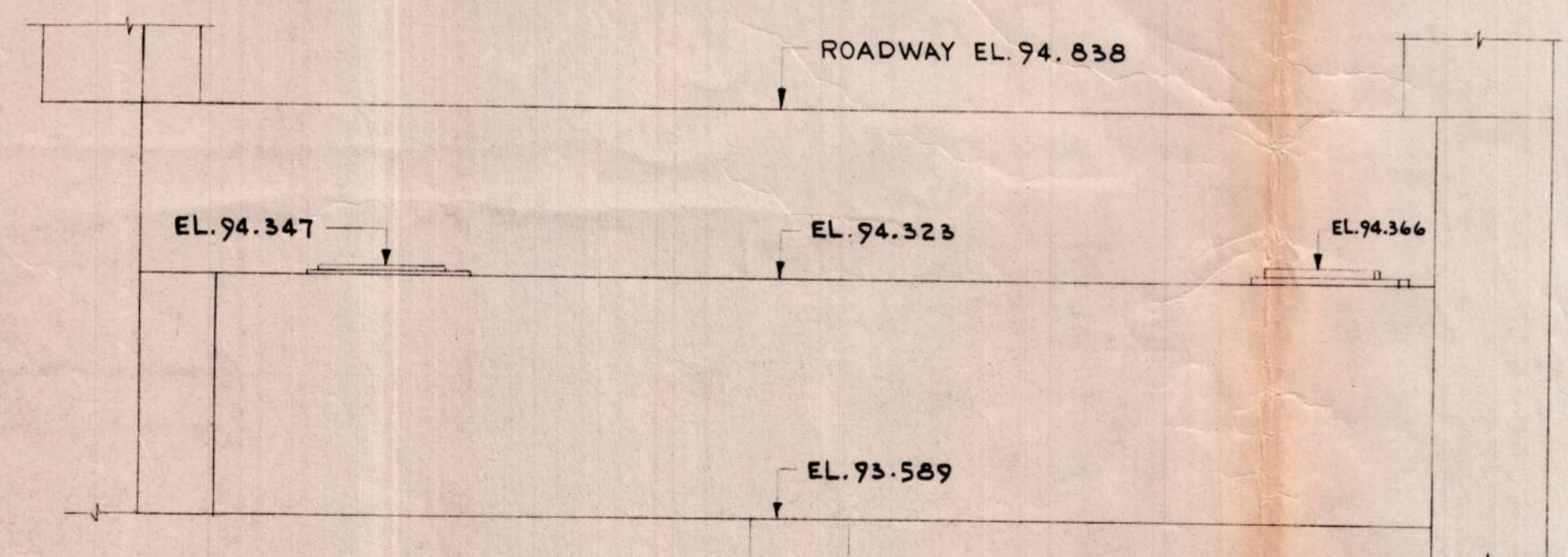
ELEVATION B-B SCALE: 1:20
