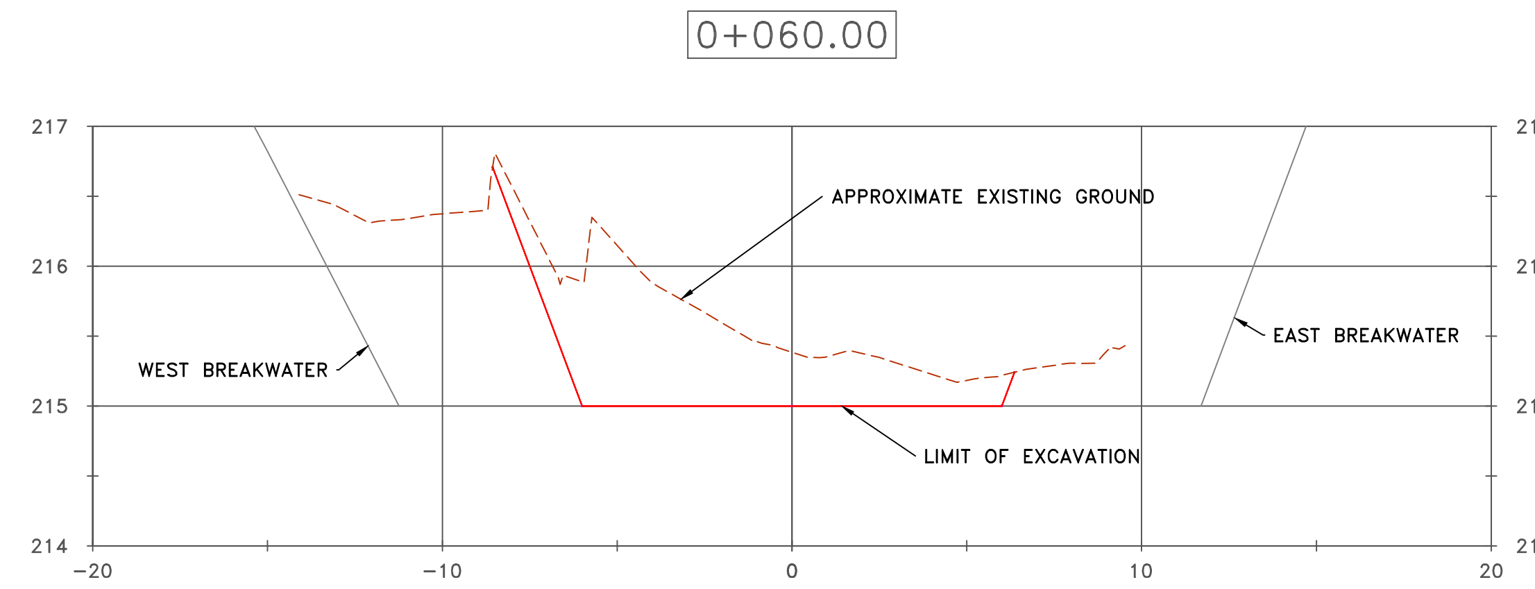
SECTION VIEWS SCALE: 1:150
