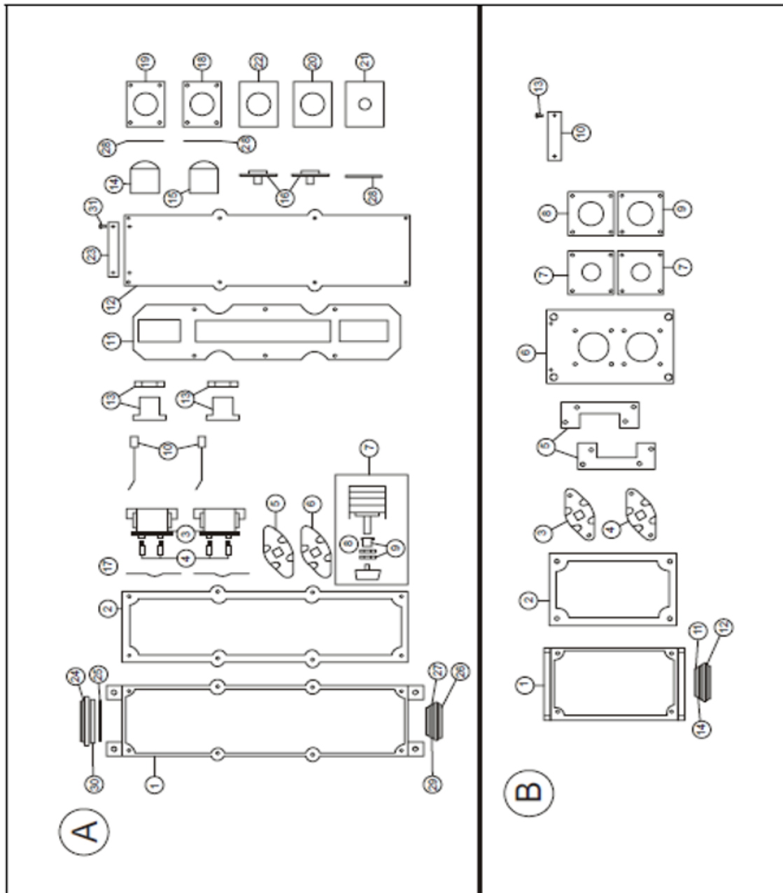
Figure 6-22 (Sheet 1 of 4) Pushbuttons and Switch Units Figure 6-22 (feuille 1 de 4) Boutons-poussoirs et commutateurs
