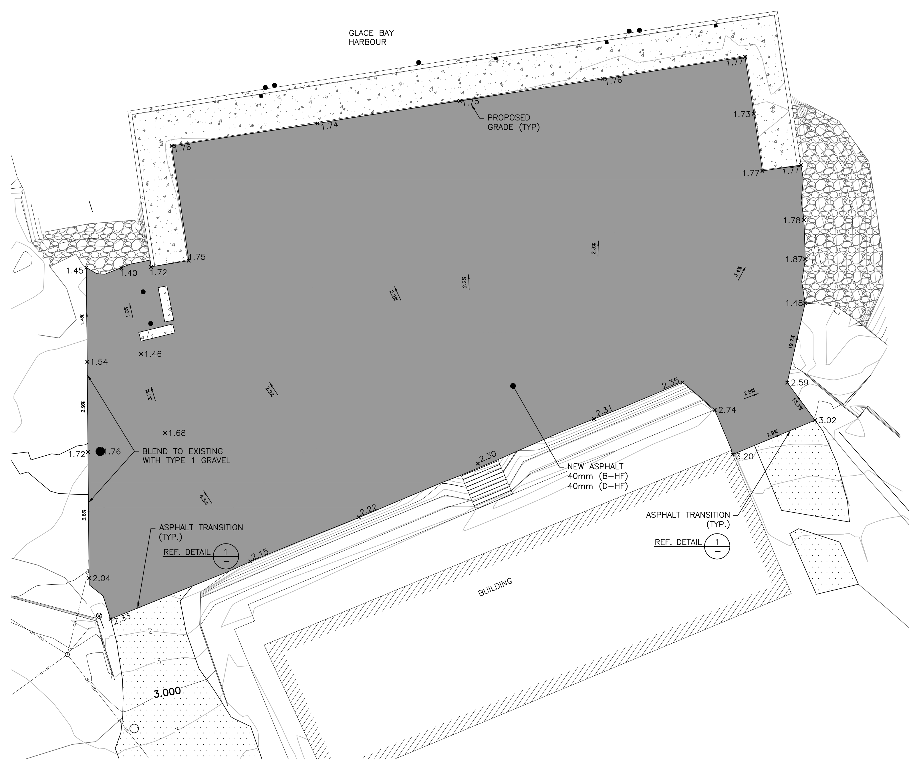
PLAN - GRADING SCALE : 1:150
