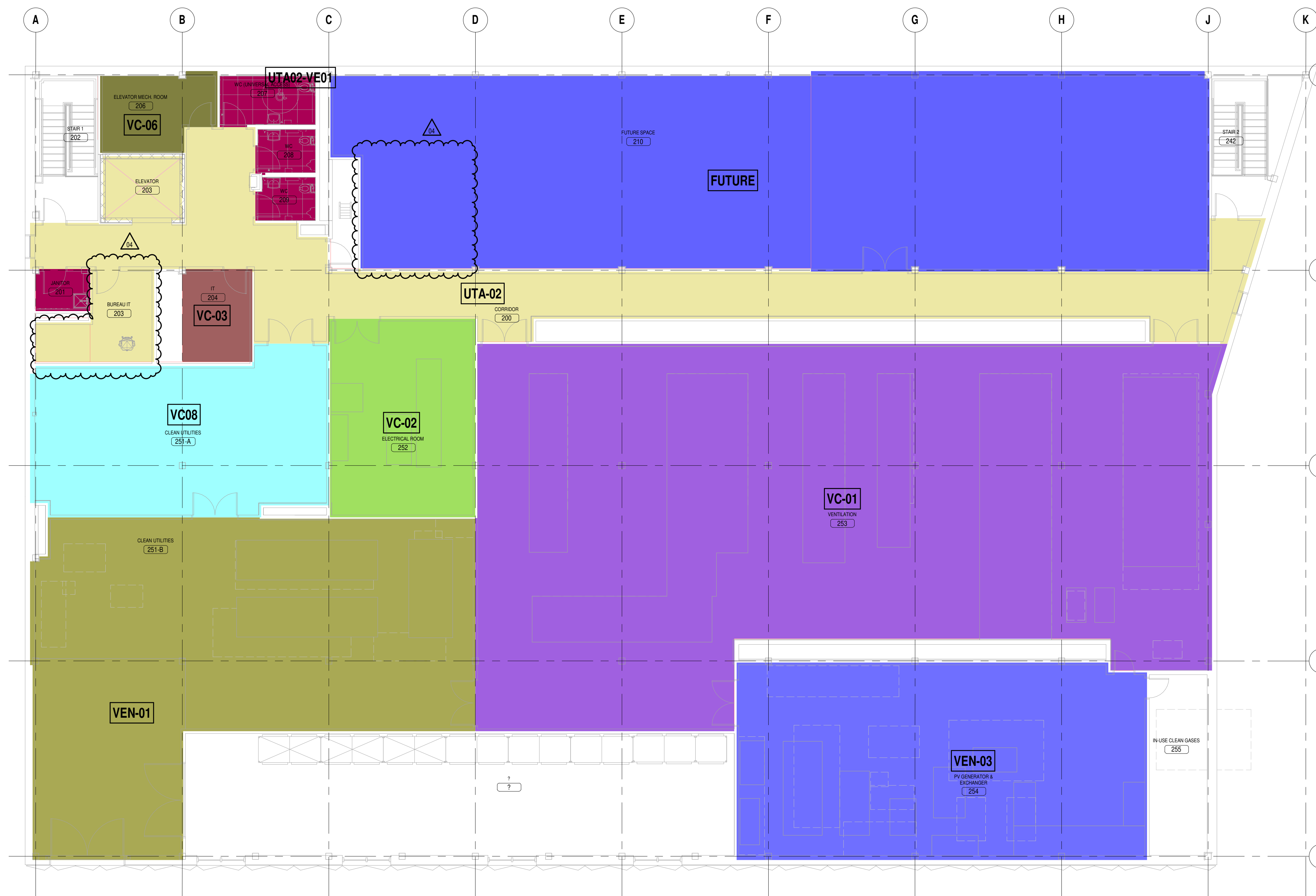
2 2e ÉTAGE - ZONAGE 1 : 100
